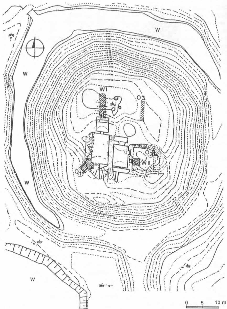
Ilustr. 2. Białaczów, stan. 3, gm. Białaczów. Plan warstwicowy kopca podworskiego z zaznaczeniem relikwów murowanego budynku WI, WII – wykopy archeologiczne, O1, O2, O3 – odkrywki archeologiczno-architektoniczne. Zasięg wykopów i odkrywek zaznaczono szrafowaniem ///
