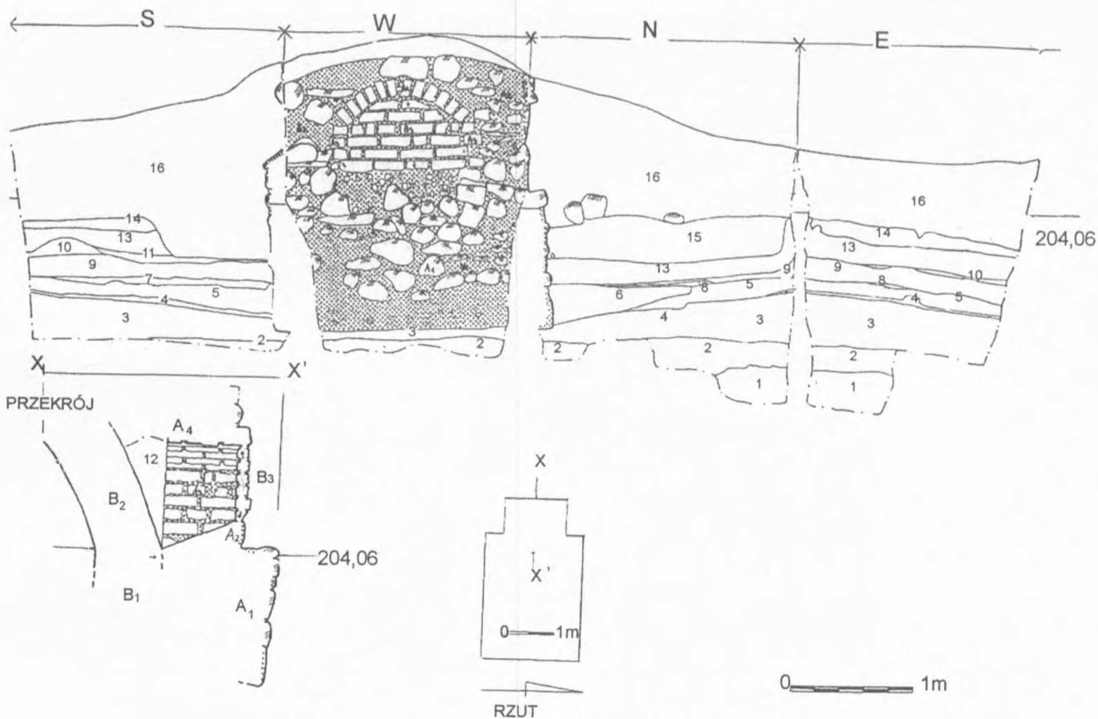
Ilustr. 5. Białaczów, stan. 3, gm. Białaczów. Wykop II – profile południowy, zachodni, północny, wschodni; przekrój X-X'; rzut wykopu A 1 – mur z łamanego piaskowca i kamieni polnych spojenych zaprawą wapienną, A 2 – mur jak wyżej, pozbawiony lica, A 3 – węgary otworu okiennego pierwotnego w murze, wykonane z cegły sztrycharskiej łączonej zaprawą wapienną, A 4 – nadproże otworu A 3 materiał jak w A 2 , B 1 – mur z łamanego piaskowca łączonego zaprawą wapienną – węzłowie sklepienia B 2 , B 2 – sklepienie z łamanego piaskowca i cegły sztrycharskiej, łączonych zaprawą wapienną, B 3 – zamurowanie otworu A 3 w murze A, wykonane z cegły sztrycharskiej, łączonej zaprawą wapienną, 1 – żółty piasek – calec, 2 – żółty piasek z przemyciami szarobrązowej próchnicy, 3 – szarobrązowa próchnica – humus pierwotny, 4 – polepa, 5 – szaroczarna próchnica z wtrętami żółtej gliny, 6 – żółta glina z wtrętami szarej próchnicy, 7 – biały piasek, 8 – rozkruszona zaprawa wapienna, 9 – szarżółta próchnica z piaskiem, dużą ilością okruchów cegły i zaprawy wapiennej oraz śladami węgla drzewnych, 10 – biały piasek z wtrętami węgla drzewnych, 11 – węgle drzewne, 12 – brunatna gliniasta próchnica z okruchami cegły i zaprawy wapiennej oraz okrzeskami łamanego piaskowca, 13 – szara, silnie spiaszczona próchnica z domieszką gliny oraz nielicznymi okruchami cegły i węglami drzewnymi, 14 – zaprawa wapienna z nielicznymi okruchami cegły, 15 – szara silnie spiaszczona próchnica z nielicznymi okruchami cegły i węglami drzewnymi, 16 – szara silnie spiaszczona próchnica z dużą ilością kamieni polnych i blokami łamanego piaskowca
