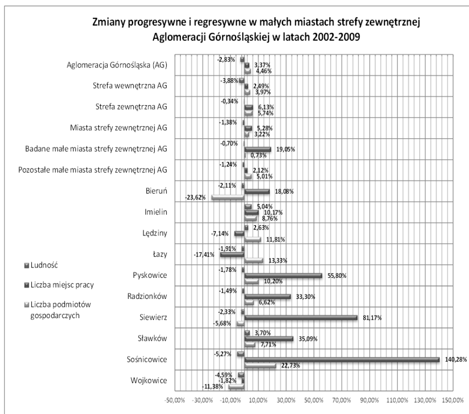
Rys. 2. Zmiany progresywne i regresywne w małych miastach strefy zewnętrznej Aglomeracji Górnośląskiej w latach 2002–2009
