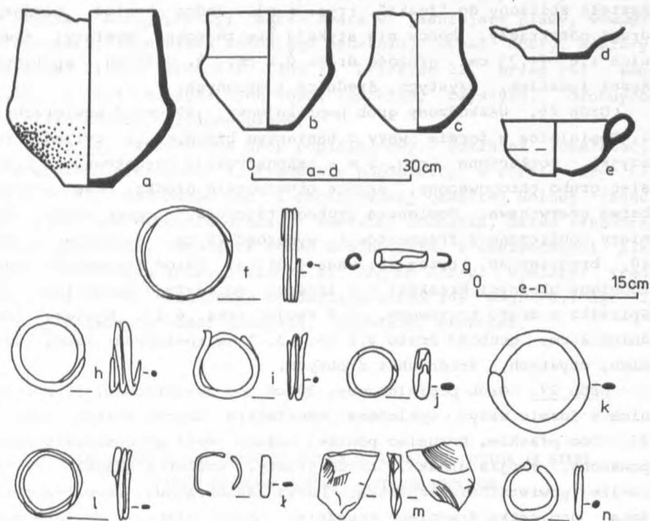
Rys. 6. Stara, gm. Aleksandrów, woj. Piotrków Trybunalski. Ceramika (a-e), zabytki brązowe (f-l, n), odłupek krzemienisty (m) z obiektów: 30 - a, 31 - b, 32 - c, 33 - d, 10 - e, 6 - f, 12 - g, 13 - h, 17 - i, 18 - j, 19 - k, 29 - l, 22 - m, 27 - m, 28 - n
