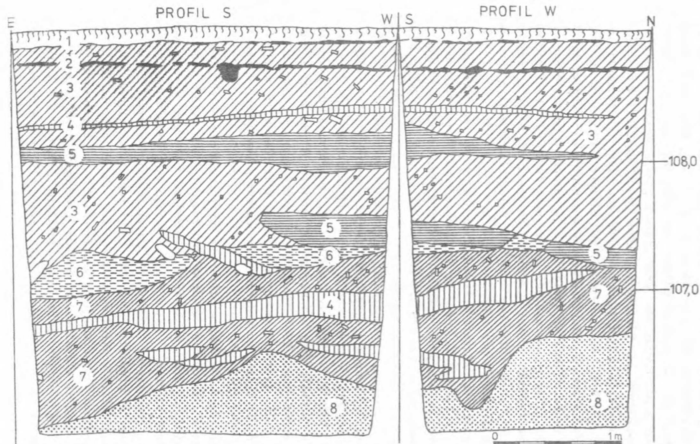
Rys. 2. Radziejów. Wykop I, profile S i W. 1 - próchnica współczesna, 2 - żużel, 3 - próchnica gliniasta z węglami drzewnymi, ułamkami cegły, gliną i zaprawą, 4 - żółty piasek podsypkowy, 5 - próchnica z piaskiem i gliną, 6 - glina, 7 - ciemna próchnica gliniasta z piaskiem, węglami drzewnymi i ułamkami cegły i grudkami polepy, 8 - piasek żółty calcowy. Rys. M. Cyrek
