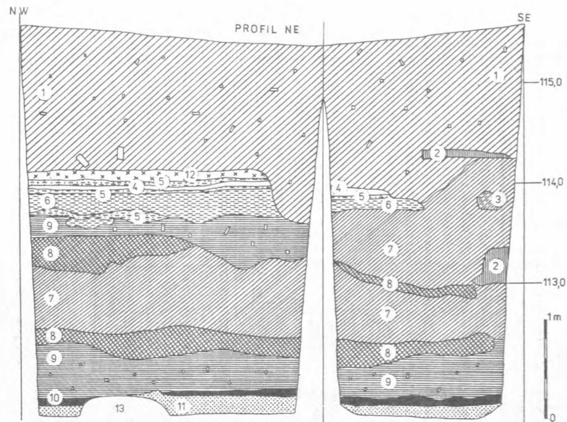
Rys. 4. Radziejów. Wykop III, profile N i E. 1 - szarobrunatna próchnica z węglami drzewnymi, ułankami cegieł, gliną i zaprawą wapienną, 2 - piasek żółty, 3 - żółta glina nasypowa, 4 - czarna próchnica z gliną i dużą domieszką węgla drzewnych, 5 - żółty piasek z gliną, 6 - żółta glina, 7 - ciemna próchnica z piaskiem i węglem drzewnym, 8 - żółtobrunatna glina (rozblasowane ściany budynków?), 9 - ciemnobrunatna próchnica z węglami drzewnymi, 10 - czarna próchnica nasycona węglami drzewnymi (poziom spalenizny), 11 - żółty piasek calcowy, 12 - polepa z węglem drzewnym, 13 - kamień eratyczny, Rys. M. Cyrek
