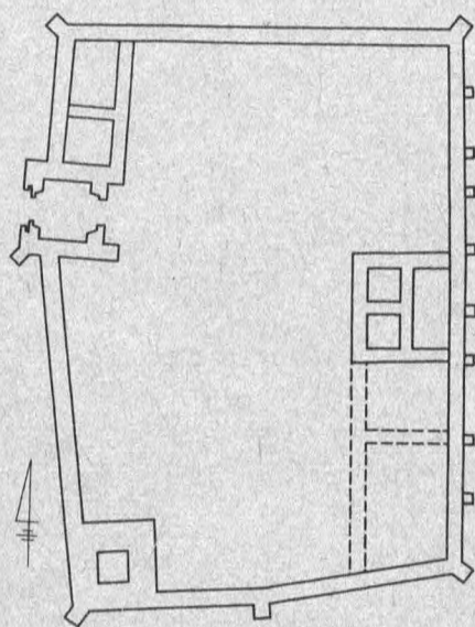
1. Łęczyca, zamek. Plan fazy kazimierzowskiej według T. Pokiewski, A. Wierstakow, E. Grabarczyk, "Dom Stary" na zamku w Łęczycy, [w:] Zamki środkowopolskie ; 2. Łęczyca, zamek. Plan po rozbudowie w połowie XVI w., ibidem
