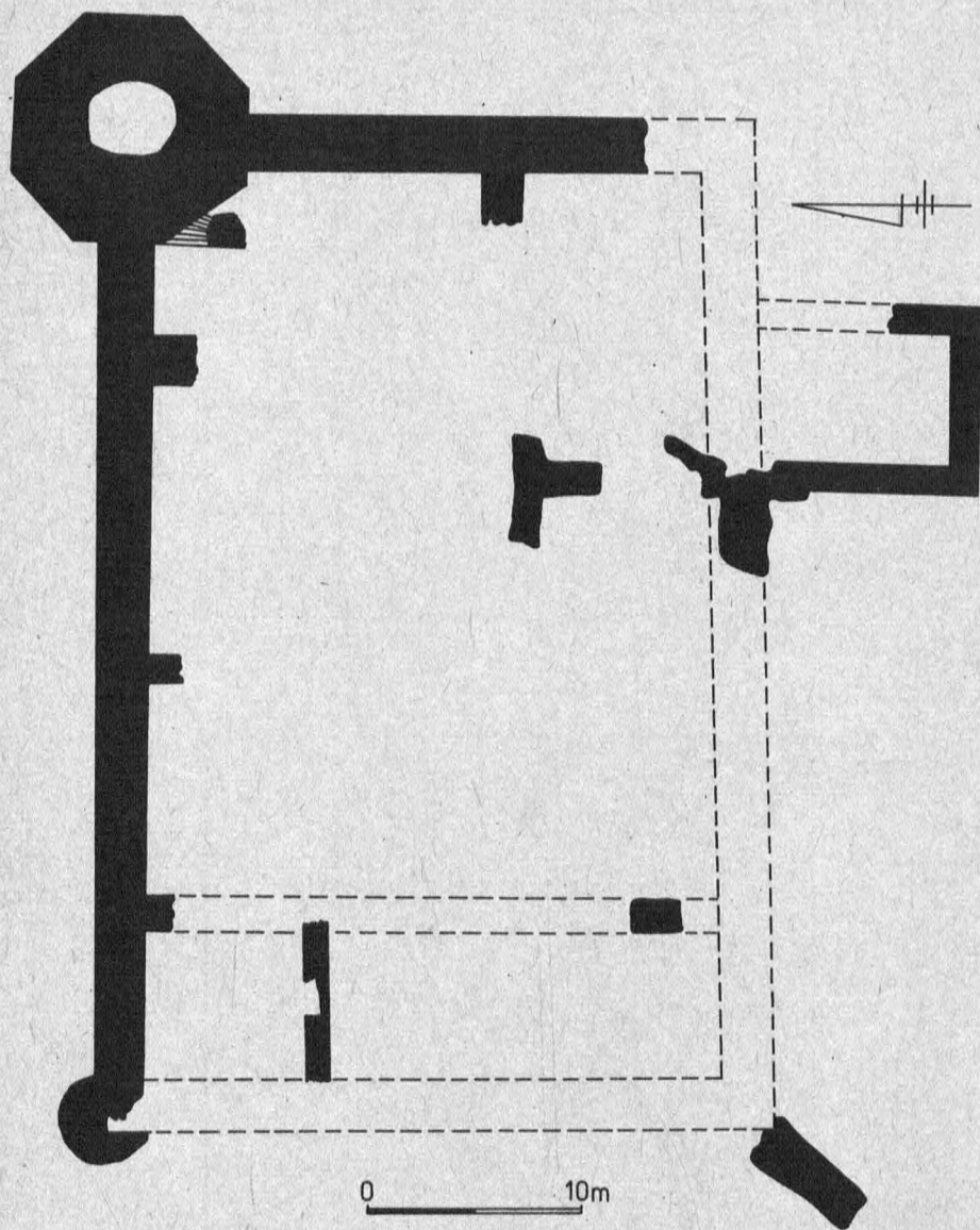
Inowłódz, zamek. Plan według J. Augustyniak, Inowłódz, IA, Badania rok 1978, w druku
