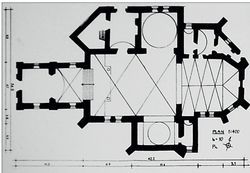
2. Kościół parafialny w Małogoszczu, rzut przyziemia
