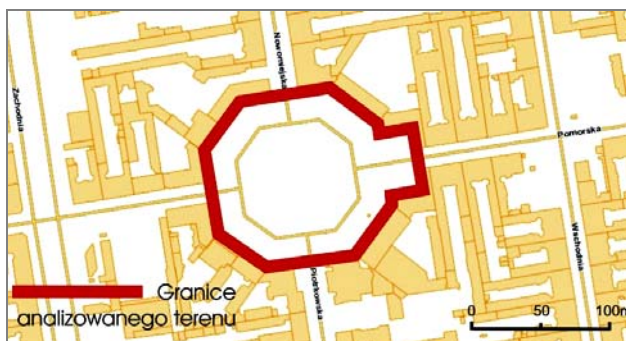
Rys. 6. Plac Wolności
