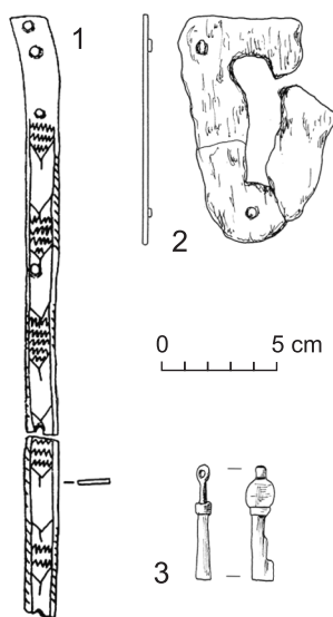
Ryc. V.11. Okucia: Jeziorsko: 1 – wykonane z brązu, Wg E. Krause, Średniowieczny gródek rycerski w Jeziorsku koło Turku , PiMMAiEwŁ, 1976, nr 23, tab. X, s. 320; Orenice: 2 – okucie dziurki klucza, 3 – kluczyk szkatułki (?). Wg M. Kołaczyk, Gródek stożkowaty w Orenicach, gm. Piątek, woj. plockie w świetle badań z lat 1986–1987 , Łódź 1990 [mps pracy magisterskiej w archiwum IA UŁ], tab. VII, VIII
