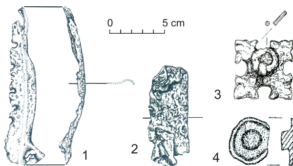
Ryc. V.10. Fragmenty brązowych okuć: 1, 2 – wg J. Górecki, M. Łastowiecki, J. Wrzesiński, Gródek na Ledniczce... , ryc. 10, s. 208; 3 – ozdobne okucie/uchwyt. Wg M. Kociński, Późnośredniowieczna siedziba obronna... , tab. XXVI; 4 – żelazny ozdobny nit. Wg M. Troszczyńska, Późnośredniowieczna siedziba obronna w Barłogach, gm. Rzgów, powiat koniński, województwo wielkopolskie, w świetle badań archeologicznych , Łódź 2007 [mps pracy magisterskiej w archiwum IA UŁ], tab. XXI
