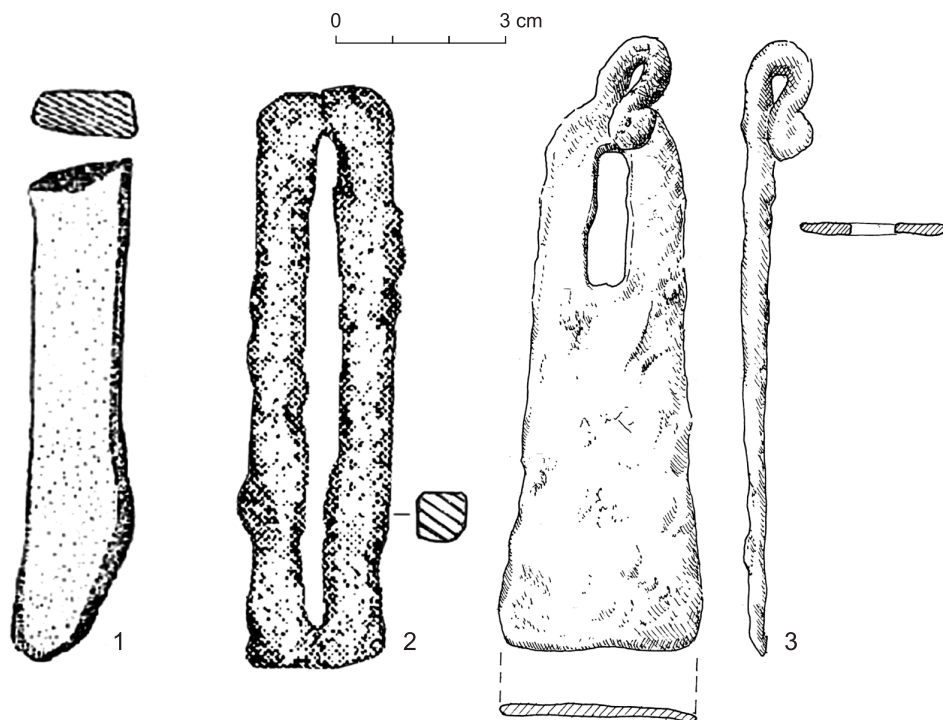
Ryc. V.28. 1 – Orłów: oselka. Wg L. Kajzer, Średniowieczny drewniany dwór obronny w Orłowie... , ryc. 17, s. 263; 2 – Barłogi: krzesiwo. Wg M. Troszczyńska, Późnośredniowieczna siedziba obronna w Barłogach... , tab. XXII; 3 – Kozłów: krzesiwo. Wg S. Kołodziejskiego
