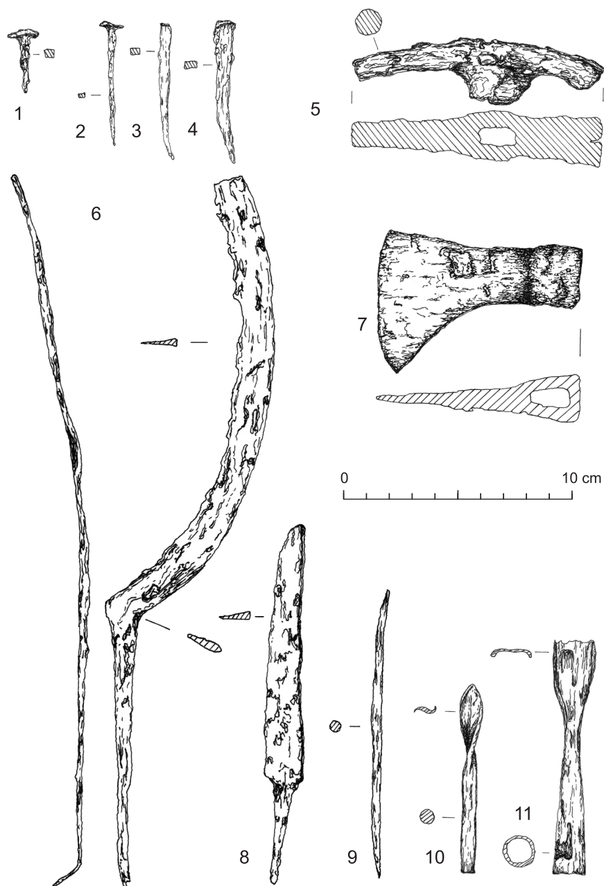
Ryc. V.23. Trzemesze: narzędzia: 1-4 – gwoździe, 5 – młotek, 6 – sierp, 7 – siekiera, 8 – nóż, 9 – szydło, 10 – świder, 11 – dłuto. Wg M. Kociński, Późnośredniowieczna siedziba obronna w Trzemeszach... , tab. XXVI
