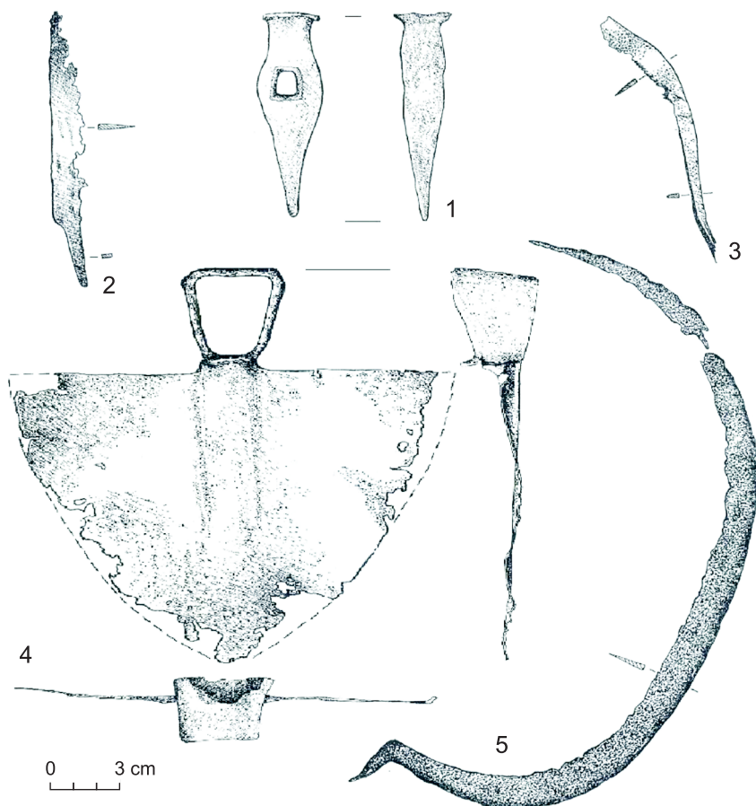
Ryc. V.20. Krzykawka: narzędzia: 1 – młotek, 2 – nóż, 3, 5 – fragmenty sierpów, 4 – kopaczka. Wg E. Szydłowska, Średniowieczny gródek w Krzykawce... , rys. 3, 4, s. 144, 145
