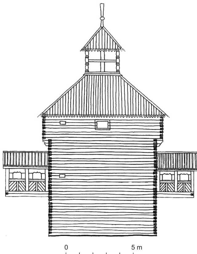
Ryc. VII.46. Zachodnia baszta twierdzy Jakuckiej, datowana na XVII w. – rekonstrukcja wg Н. П. Крадин, Русское деревянное... , гус. 196, s. 165
