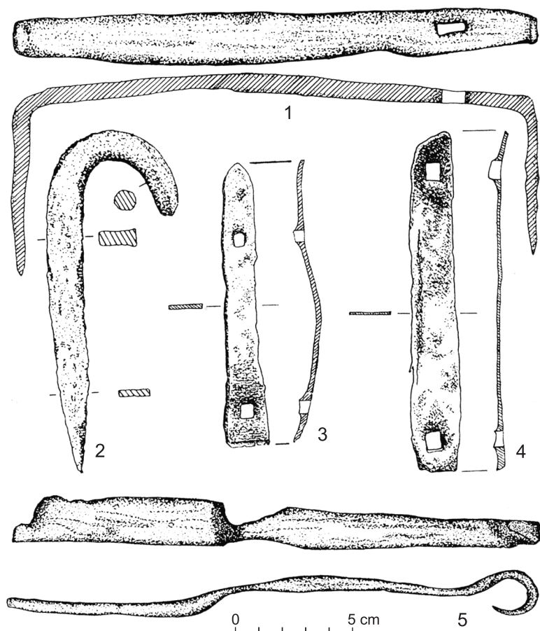
Ryc. V.9. Krzykawka. Przedmioty związane z budownictwem: 1 – klamra ciesielska, 2 – hak, 3 i 4 – okucia, 5 – zawias. Wg E. Szydłowska, Średniowieczny gród w Krzykawce... , rys. 7, s. 153
