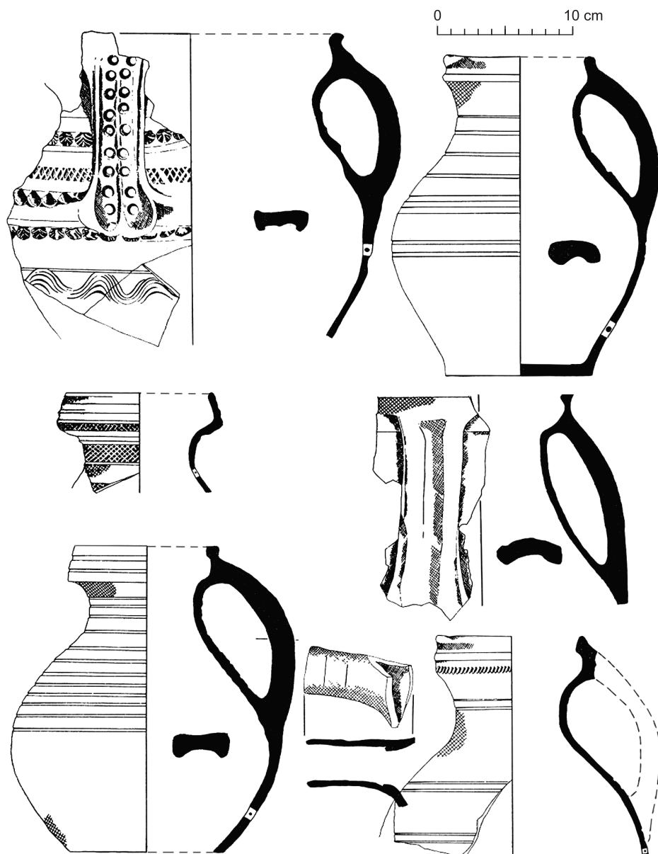
Ryc. V.15. Orłów: naczynia ceramiczne. Wg L. Kajzer, Średniowieczny drewniany dwór obronny w Orłowie... , ryc. 12, 13, s. 254
