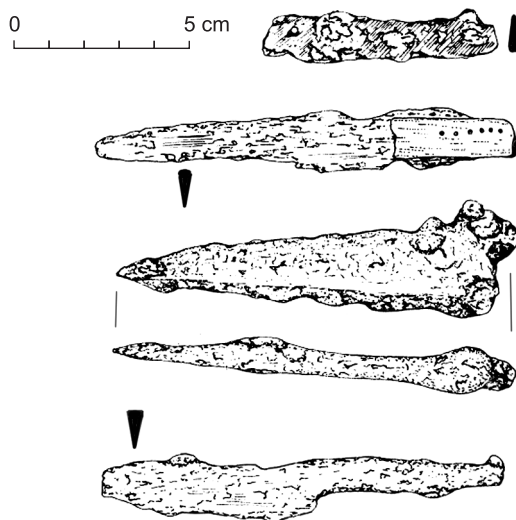
Ryc. V.26. Orłów: noże. Wg L. Kajzer, Średniowieczny drewniany dwór obronny w Orłowie... , ryc. 16, s. 262
