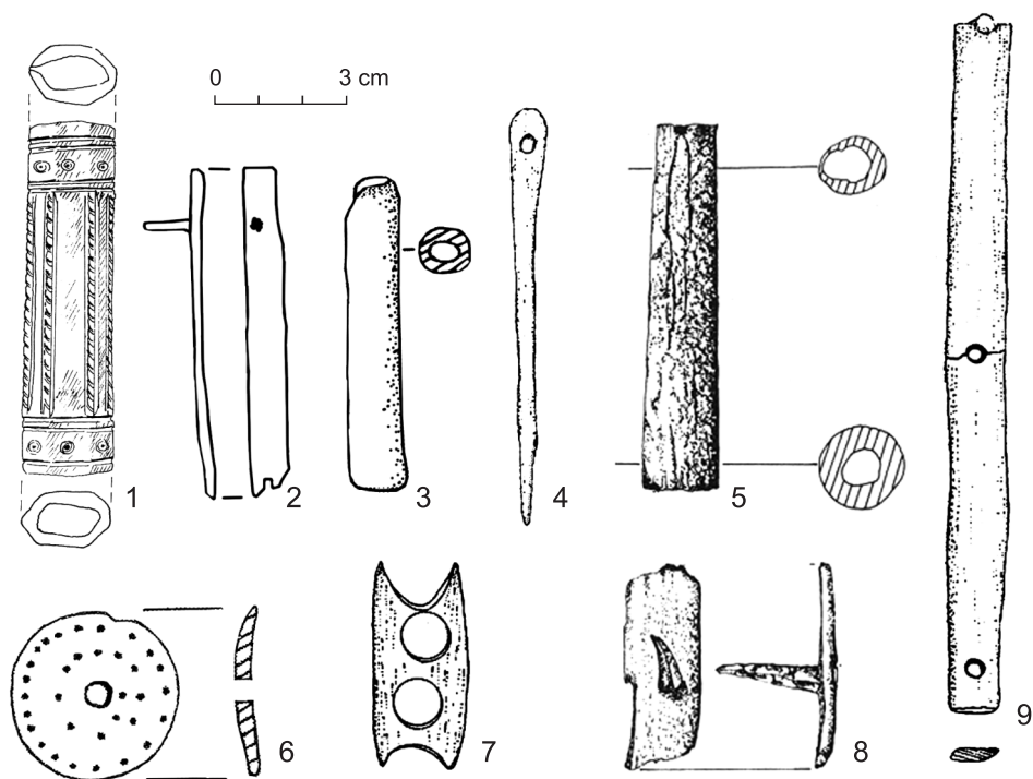
Ryc. V.27. Przedmioty kościane: Kozłów: 1 – oprawka. Wg S. Kołodziejskiego: Barłogi: 2 – okładzina, 3 – rurka, 6 – płytką z ornamentem. Wg M. Troszczyńska, Późnośredniowieczna siedziba obronna w Barłogach... , tab. XXIV; Orlów: 4 – szydło, 7 – półprodukt, 9 – okładzina. Wg L. Kajzer, Średniowieczny drewniany dwór obronny w Orlowie... , ryc. 17, s. 263; Ledniczka: 5 – oprawka kościana, 8 – fragment okładziny z poroża z nitom z tego samego materiału. Wg J. Górecki, M. Łastowiecki, J. Wrzesiński, Gródek na Lednicze... , ryc. 10, s. 208
