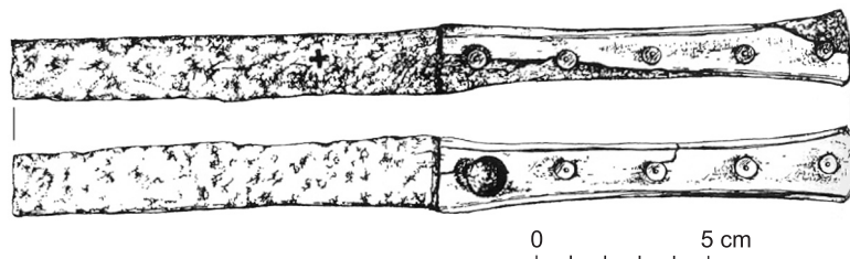
Ryc. V.24. Ledniczka: nóż. Wg J. Górecki, M. Łastowiecki, J. Wrzesiński, Gródek na Lednicze... , ryc. 12, s. 212
