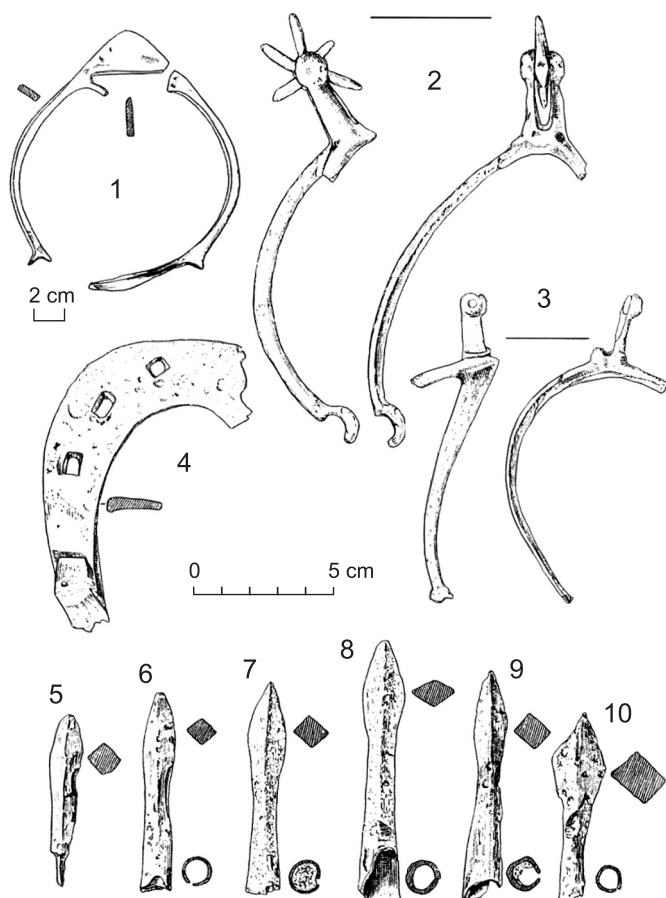
Ryc. V.32. Rozprza: militaria: 1 – strzemię, 2–3 – ostrogi, 4 – podkova, 5–10 – groty beltów. Wg A. Chmielowska, Rozprza we wczesnym i późnym średniowieczu... , tab. VI, s. 205
