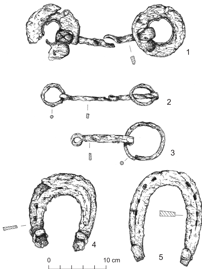
Ryc. V.36. Trzemsze: 1–3 – wędzidła, 4–5 – podkowry. Wg M. Kociński, Późnośredniowieczna siedziba obronna w Trzemszach... , tab. XXII
