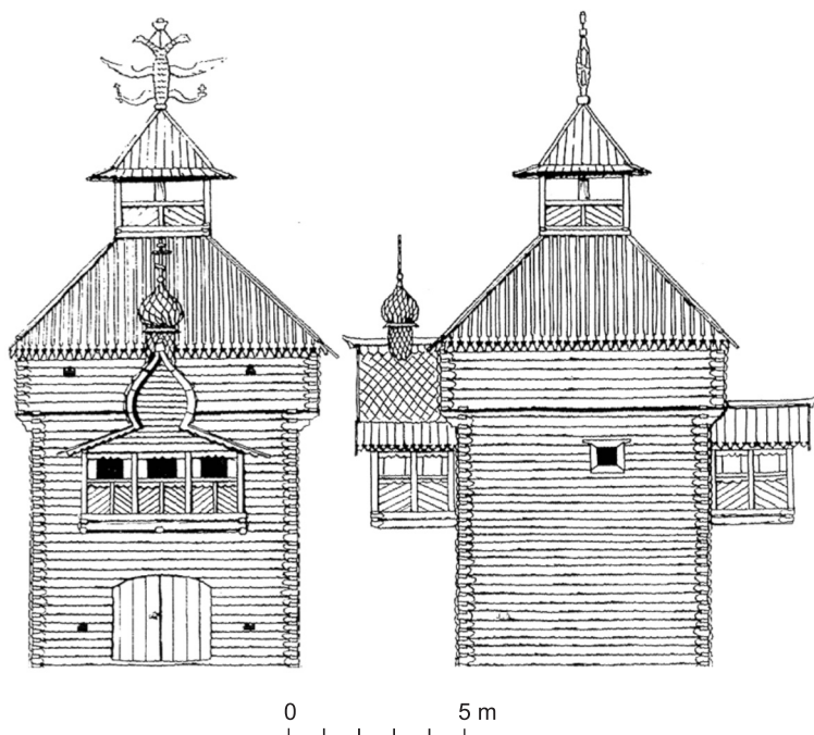
Ryc. VII.45. Baszta obronnego miasta Ilmsk na Syberii, rekonstrukcja wg H. П. Крадин, Русское деревянное оборонное зодчество , Москва 1988, s. 111
