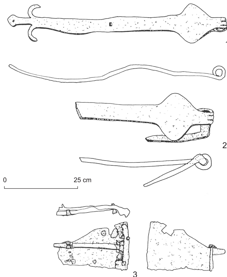
Ryc. V.2. Żelazne elementy drzwi: 1, 2 – okucia; 3 – zamek. Wg J. Pierzak, D. Rozmus, Gródek rycerski w Kozłowie... , ryc. 8, s. 30
