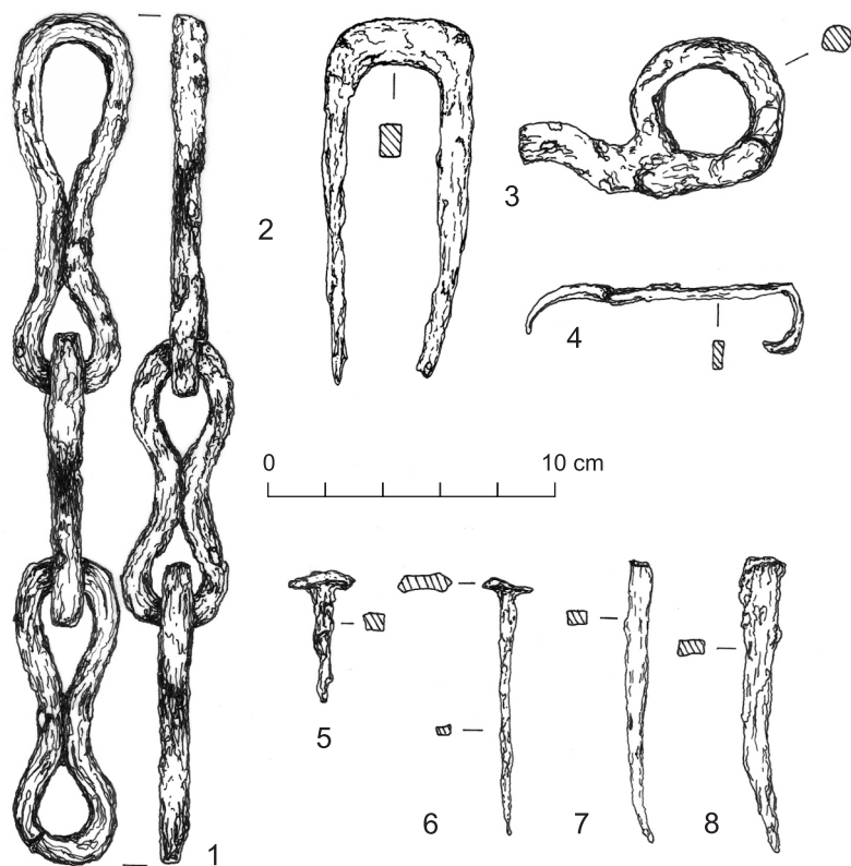
Ryc. V.3. Trzemsze: 1 – wrzęciadź, 2 – skobel, 3, 4 – klamry budowlane (?), 5–8 – gwoździe. Wg M. Kociński, Późnośredniowieczna siedziba obronna w Trzemszach w woj. konińskim , Łódź 1995 [mps pracy magisterskiej w archiwum IA UŁ], tab. XXIV, XXV
