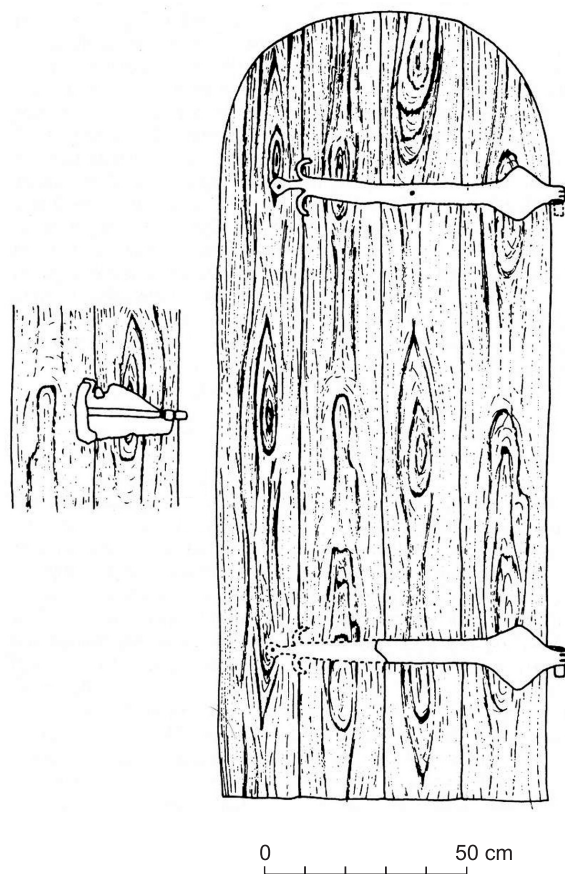
Ryc. V.1. Rekonstrukcja drzwi na podstawie znalezisk z Kozłowa gm. Sośnicowice. Wg J. Pierzak, D. Rozmus, Gródek rycerski w Kozłowie, gm. Sośnicowice , „Rocznik Muzeum w Gliwicach” 1997, t. 11/13, ryc. 9, s. 31
