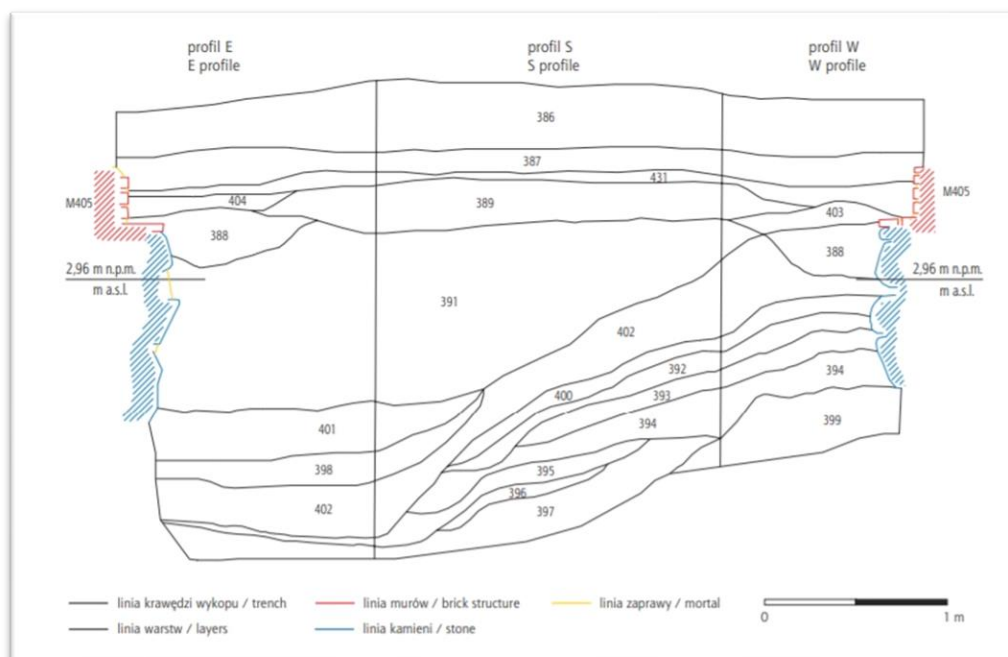
Ryc.6.74 Profil sondażu 13 z 2013 roku. Nasyp wału Szańca Wschodniego tworzą warstwy 397 -402, warstwa 391 to niwelacja podnosząca teren przecięta przez wkop pod mur Kościoła św. Olafa (W.388, 403), poziom budowlany obiektu tworzą warstwy 389,431, z rozbiórką kościoła można wiązać w. 386,387. ( rys. M. Nowak, A. Kołodziejczyk oprac. J. Dąbał, w: Dąbał 2015, s. 114)
