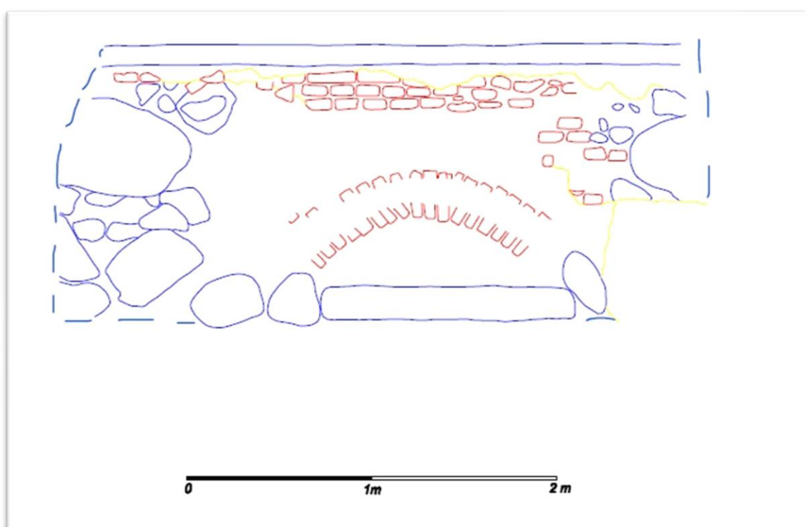
Ryc.6.14 Fragment zachodniego lica kurtyny zachodniej z widocznym sklepionym otworem ściekowym.
