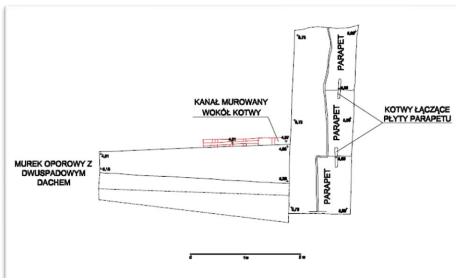
Ryc.6.17 C -rzut korony muru wschodniego i przypory ( rys. B. Balewska, oprac. M. Schmidt)
