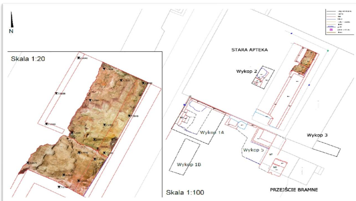
Ryc.3.57 Rzut budynku Starej Apteki z odsłoniętym fragmentem gotyckiej baszty na współczesnym planie miasta (pomiar i oprac. P. Muntowski)
