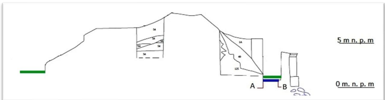
Ryc.6.19 Przekrój przez wał południowy Fortu Carre. Kolorem zielonym oznaczono współczesny poziom użytkowy fosbrei i dziedzińca fortu, kolorem niebieskim oznaczono XVII -XX wieczny poziom użytkowy fosbrei, A - fundament przypory zabezpieczającej przed osuwaniem nasyp, B - Fundament muru fosbrei (rys. B. Balewska, na podstawie inwentaryzacji fotogrametrycznej Holcer i inni 2005, oprac M. Schmidt)
