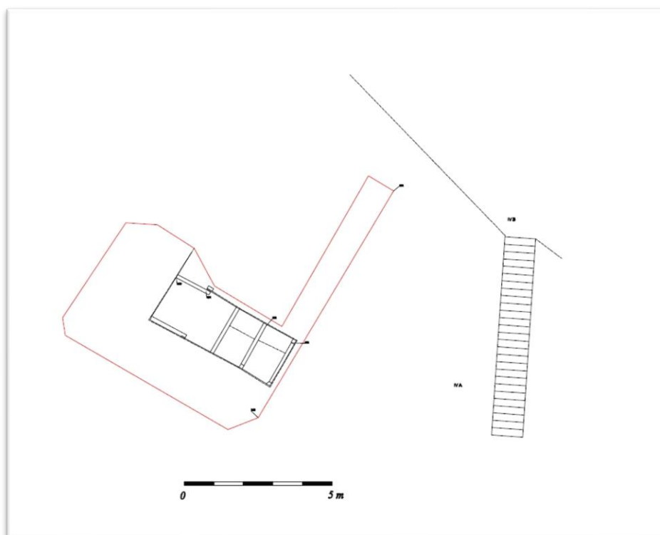
Ryc.6.21 Pozostałości drewnianej piwnicy wkopanej w wał południowy. B - ściana zachodnia i podłoga konstrukcji. Widok od E (fot. M. Kasprzak C- rzut podłogi konstrukcji (rys i oprac. P Janda)
