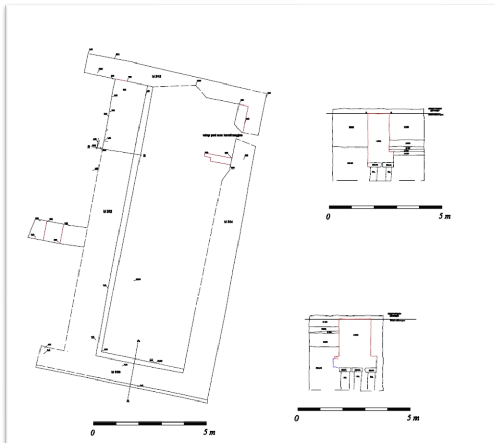
Ryc.6.71 Rzut XVIII wiecznego budynku przy wjeździe do Fortu Carre. Po prawej stronie przekroje przez fundamenty obiektu i przylegające do niego warstwy ziemne (rys. P. Janda, oprac. M. Kasprzak)
