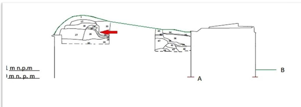
Ryc.6.16 Przekrój przez wał wzdłuż wschodniej kurtyny Fortu Carre (wykop III z 2003 roku). Kolorem zielonym oznaczono poziom użytkowy z 2003 roku, czerwona strzałką oznaczono nasyp z XVII-XVIII wieku, A poziom fundamentów koszar, B - poziom użytkowy dziedzińca Fortu Carre (rys. B. Balewska, na podstawie inwentaryzacji fotogrametrycznej Holcer i inni 2005, oprac. M. Schmidt)
