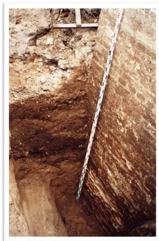
Ryc.6.30 A - Zbliżenie na mur oporowy przy poternie do bastionu Artyleryjskiego na styku z zachodnią ścianą Domu Porucznika Piechoty do, której został dostawiony. Widok od NW (fot. M. Kasprzak) B - zbliżenie na ścianę zachodnią Domu Porucznika Piechoty. Widoczna zacierka świadcząca o tym, że ściana ta była pierwotnie odsłonięta. W części dolnej widoczny fundament muru w wąsko przestrzennym wkopie
