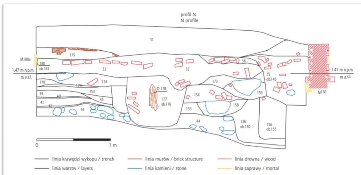
Ryc.6.42 Profil północny wykopu 2 z 2013 roku (rys. D. Leśniewska, oprac. J. Dąbał : Dąbał 2015, s.89). W profilu widoczne są XVI wieczne poziomy użytkowe (w. 39-43), pozostałości obiektów związanych z okresem budowy Fortu Carre (w. 153,154,159, 177), pozostałości najstarszego budynku (w.32,36), z kolejnym budynkiem związane były warstwa 175 oraz mur 180a, pozostałości murowanego domu z przełomu XVIII i XIX wieku ( ob. 145 i mur 150)
