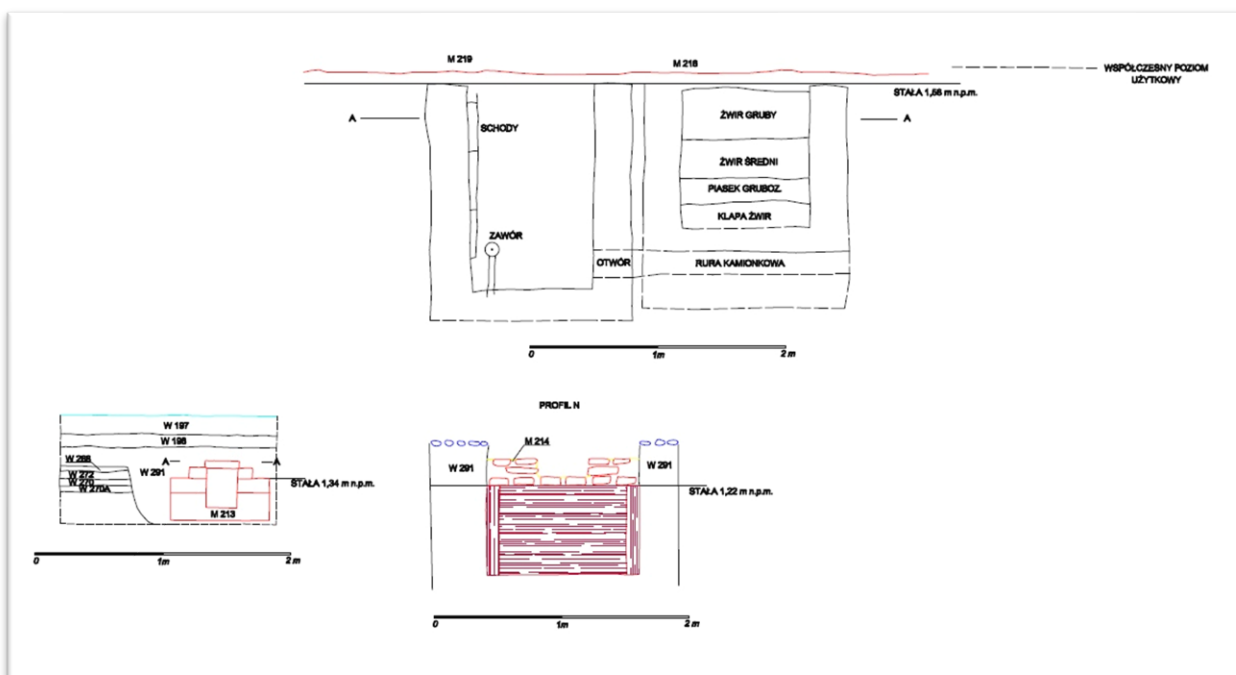
Ryc.6.64 Po lewej przekrój przez XIX w kanał burzowy, po prawej przekrój przez XIX wieczną studzienkę ściekową, u góry przekrój przez XX wieczne studzienki zlokalizowane przy nieistniejącej pompie (rys. B. Balewska, oprac. M. Kasprzak)
