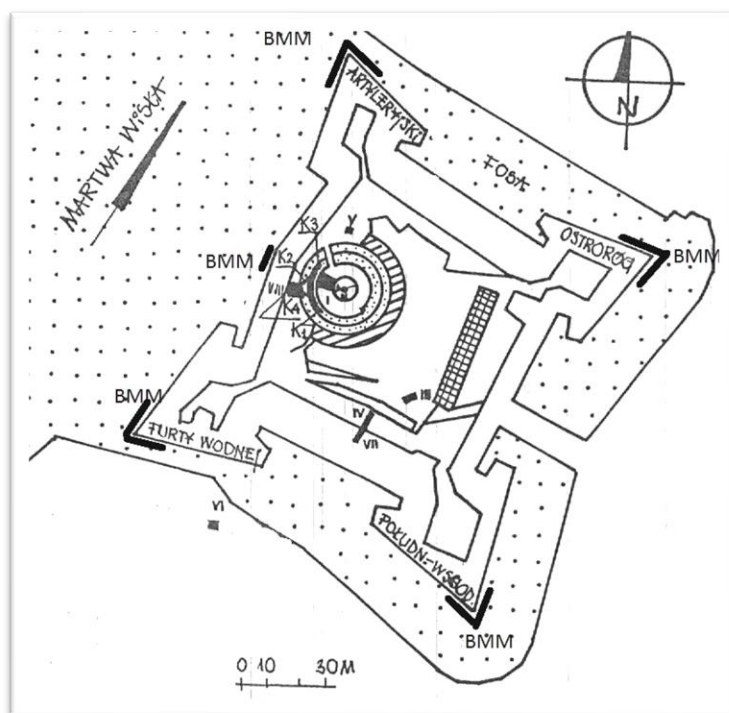
Ryc.6.3 Schematyczny plan Fortu Carre z naniesionymi wykopami archeologicznymi z lat 1968-1970 (oznaczone cyframi I -VIII) oraz badań Centralnego Muzeum Morskiego z 1993 roku (oznaczone na planie literami BMM), K1- K4 - oznaczono odcinki korytarzy w dolnej części Wieńca odkryte podczas badań archeologicznych ( Zbierski 1977, s.134, rys.1 oraz Zbierski 1999, s.51)
