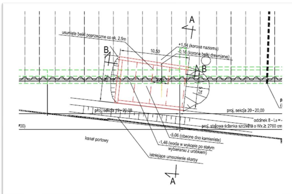
Ryc.6.75 B rzut fragmentu odsłoniętych XVII –XVIII wiecznych umocnień brzegowych wzdłuż Nabrzeża Zbożowego -sekcja 19 (Archeoscan Pracownia Archeologiczno –konserwatorska Sylwia Kurzyńska, oprac. M. Korzonek)
