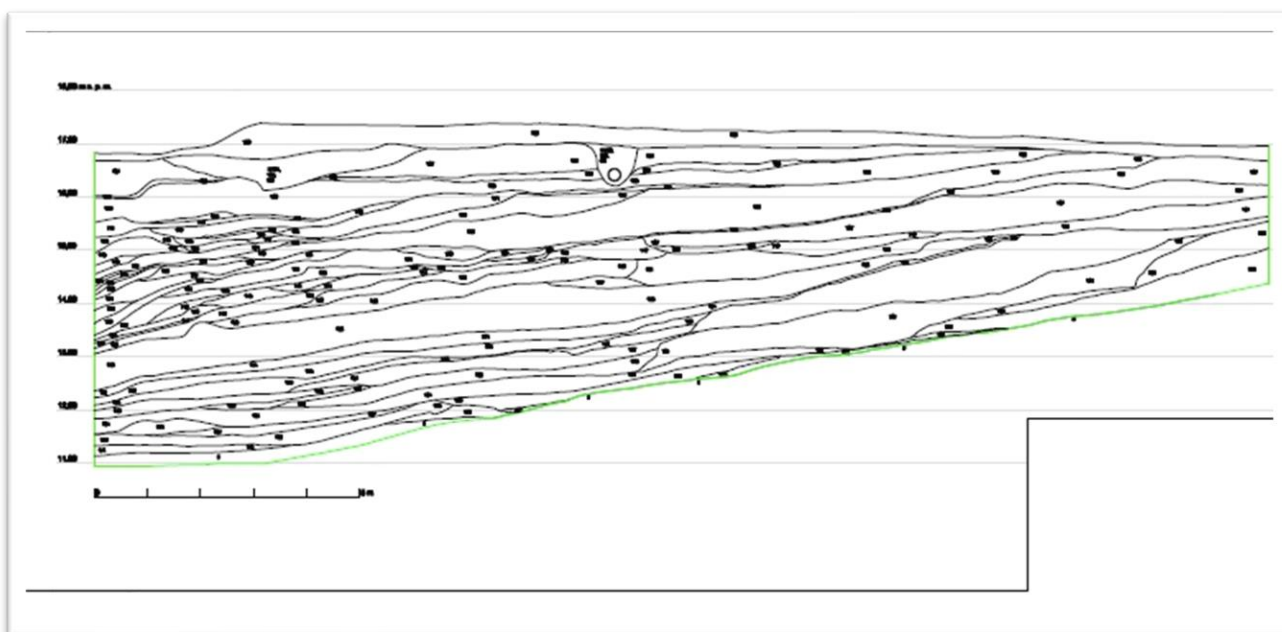
Ryc.5.59 Przekrój przez niwelacje tworzące zasyp Suchej Fosi zarejestrowanej w trakcie badań z 2010 roku przy ulicy 3 Maja 9 w wykopie 4 (rys. i oprac. P. Muntowski)
