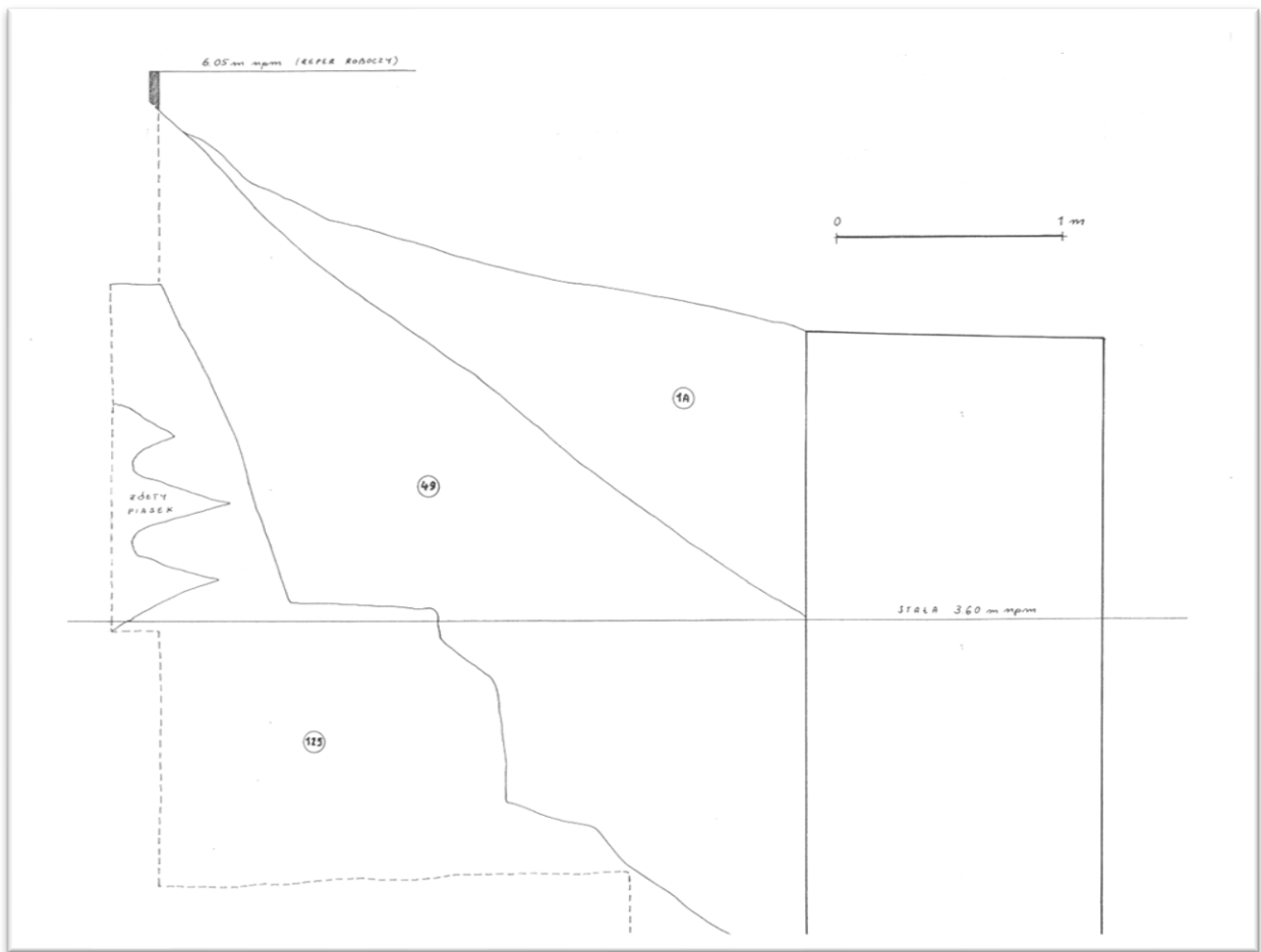
Ryc.6.18 D -Przekrój przez wykop XVIII z 2003 roku (rys. B. Balewska, oprac. M. Schmidt)
