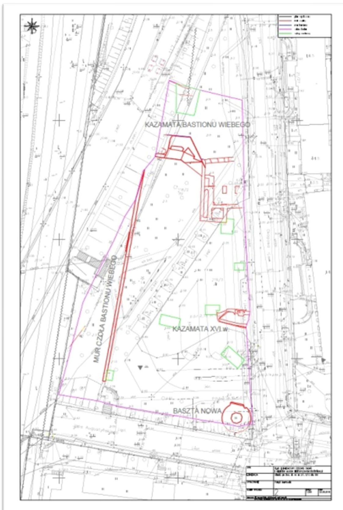
Ryc. 3.2 Ryc.II.2 Rzut odkrytych w czasie badań prowadzonych w 2018 roku relikwów późnogotyckich i nowożytnych murowanych elementów fortyfikacji na współczesnym planie do celów projektowych (oprac. P. Muntowski)
