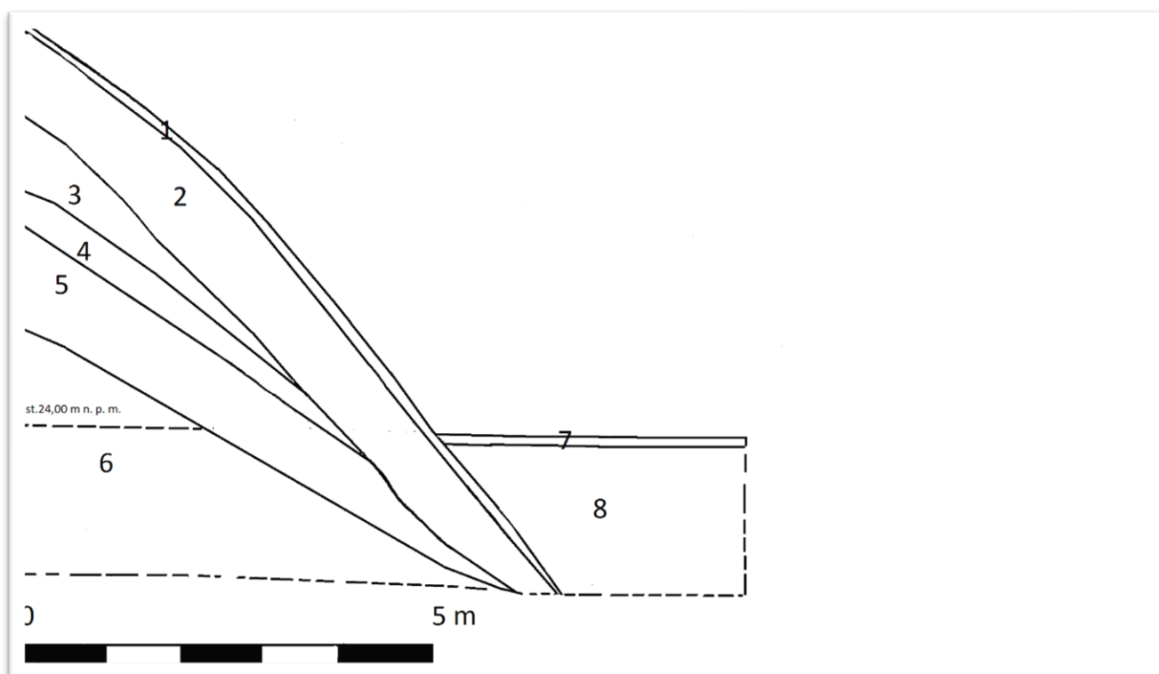
Ryc.5.9 B przekrój przez nawarstwienia w sondażu III (rys. M. Kasprzak) C -przekrój przez nawarstwienia w sondażu I (rys. M. Kasprzak)
