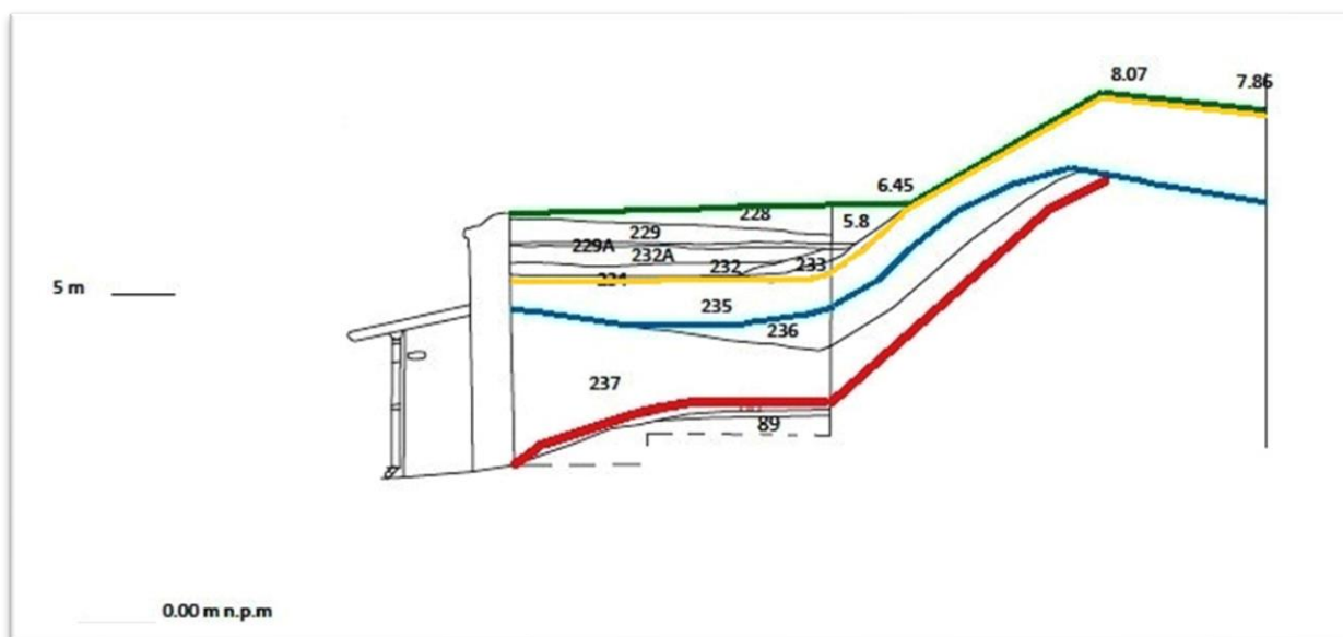
Rys.6.25 Przekrój przez wał północny Fortu Carre. Kolorem czerwonym oznaczono pierwotny kształt nasypu, kolorem niebieskim oznaczono nasyp w okresie XVII -XVIII wiek, kolorem żółtym oznaczono XIX wieczny poziom użytkowy, kolorem zielonym oznaczono współczesny poziom użytkowy. Widok od E (na podstawie inwentaryzacji fotogrametrycznej Holcer i inni 2005oprac. M. Kasprzak)
