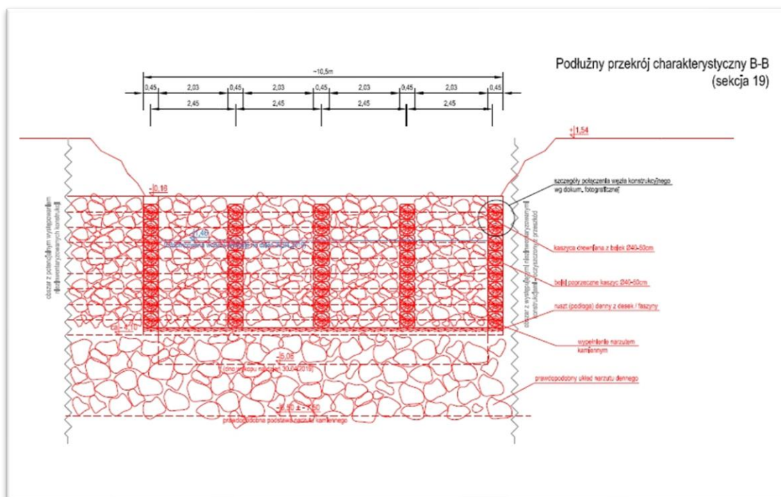
Ryc. 6.76 B przekrój podłużny B-B jednej z kaszyc (sekcja19) odkrytych wzdłuż nabrzeża Zbożowego w 2019 roku (Archeoscan Pracownia Archeologiczno –konserwatorska Sylwia Kurzyńska, oprac. M. Korzonek)
