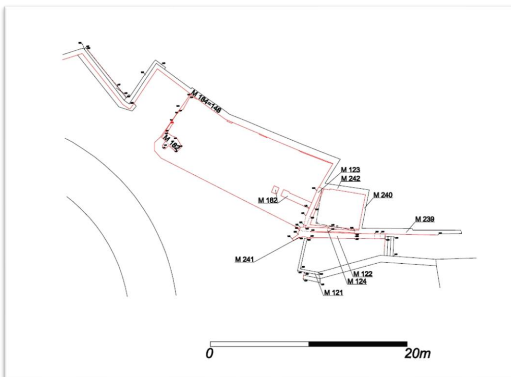
Ryc.6.34 Rzut fundamentów i zachowanych murów budynków w północnej części Fortu Carre. M 164=148 - ściana północna Domu Porucznika Piechoty, M 123 -- ściana wschodnia budynku, M 182 - ściana południowa budynku, po lewej M 182 wraz ze starszym murem, A pierwsza ściana zachodnia Domu Porucznika Piechoty, B - Druga ściana zachodnia domu, Mur 242 północna ściana kuźni, M 240 ściana zachodnia kuźni, Mur 124 ścian południowa kuźni, Mur 122 i 241 - XIX wieczna kanalizacja burzowa, M 121 - mur oporowy współczesnego podjazdu północnego (rys. P. Janda, oprac. M. Kasprzak)
