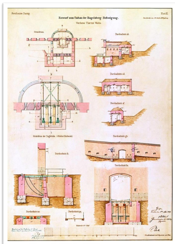
Ryc.5.40 A Projekt Bramy Północnej wraz z wartownią ze zbiorów Archiwum Państwowego w Gdańsku. B Projekt mostu zwodzonego przy bramie ze zbiorów Archiwum Państwowego w Gdańsku. Szukam źródła miałam je ze strony internetowej, której już nie ma.
