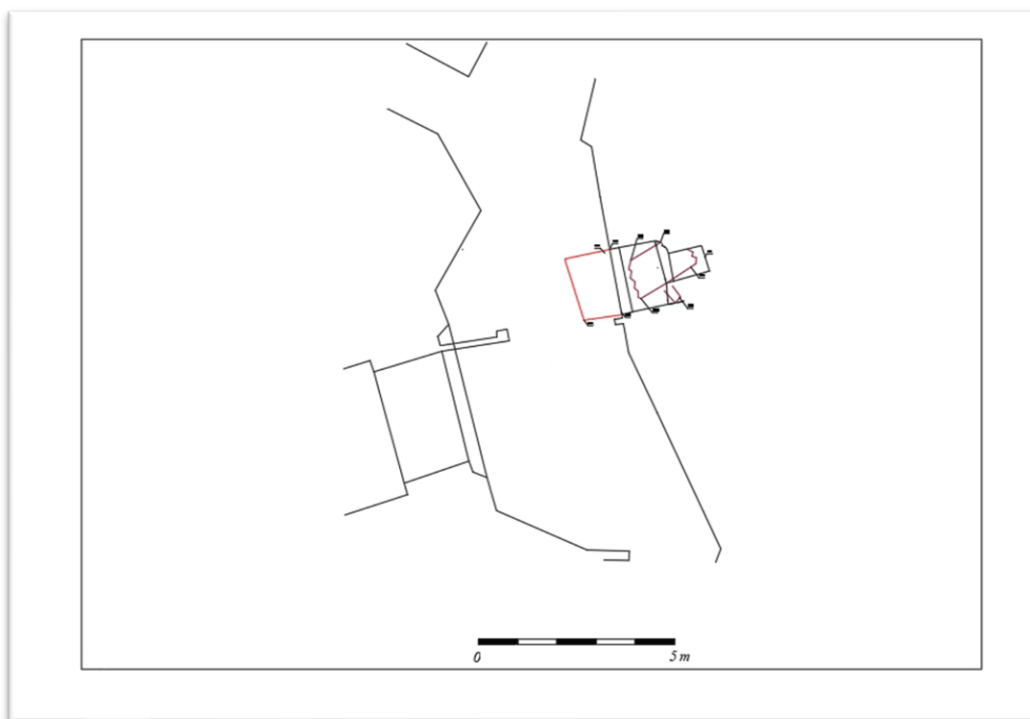
Ryc.6.47 Rzut pozostałości drewnianego obiektu - najprawdopodobniej XVI wiecznego blokhauzu odkrytego poniżej współczesnego poziomu użytkowego wewnątrz Bastionu Ostroróg (rys. P. Janda, oprac. P. Schmidt, M. Kasprzak)
