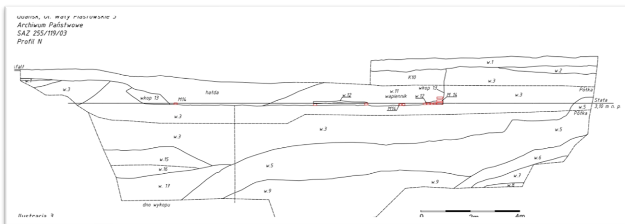
Ryc.2.18 Przekrój przez fragment późnośredniowiecznej fosy odsłoniętej w trakcie badań przy Archiwum Państwowym w Gdańsku w 2010 roku. Warstwy: w1,w2 - nawarstwienia współczesne, K 10 - konstrukcja z okresu budowy archiwum, w3 - podstawa nowożytnego wału, warstwy w5,w9, w15-17 - zasyp fosy, warstwy: w 6-8 nawarstwienia z okresu funkcjonowania fosy (rys. M. Jagusiak, oprac. Dział Cyfryzacji i Archiwizacji Muzeum Archeologiczne w Gdańsku)
