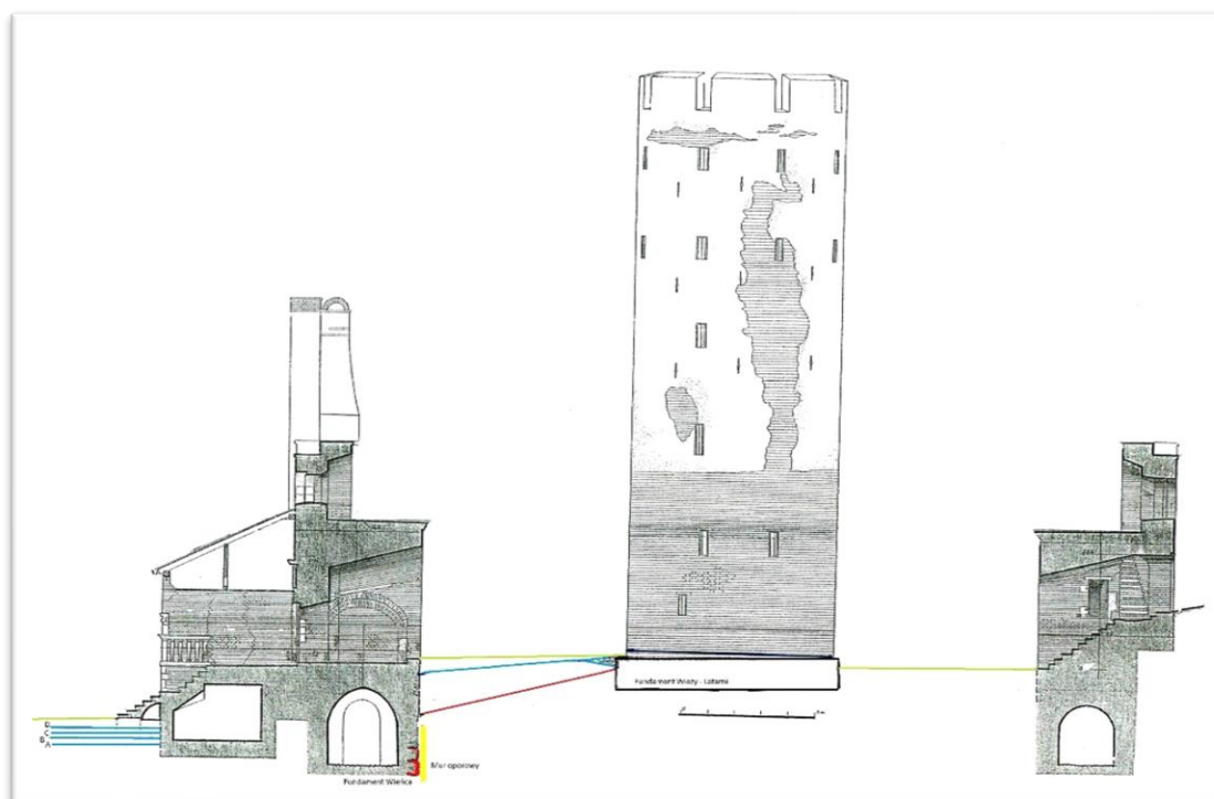
Ryc.6.4 Przekrój przez Wieżę -Latarnię i Wieńiec. Kolorem czerwonym oznaczono poziom użytkowy wokół wieży w XV wieku. Kolorem niebieskim oznaczono poziom użytkowy z okresu nowożytnego wokół wieży oraz cztery fazy poziomów użytkowych dziedzińca Fortu Carre. Kolorem zielonym oznaczono współczesny poziom użytkowy. Przekrój przez Wieżę -Latarnię i Wieńiec wykonany przez studentów Politechniki Gdańskiej – E. Nakonieczną, B. Witkowską, M. Zając, oprac. M. Kasprzak)
