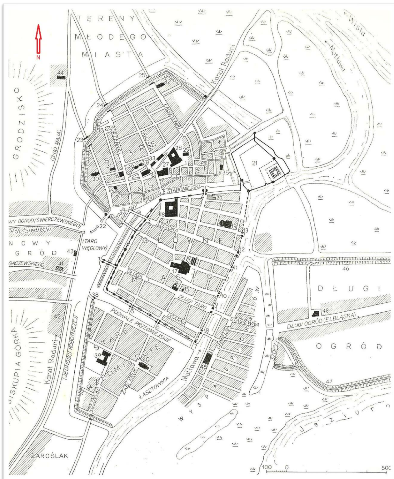
Ryc.1.5 Fortyfikacje Gdańska około 1460 roku Według R. Massalsiego i J. Stankiewicza (Kowalski, Massalski, Stankiewicz, 1969, s. 132)
