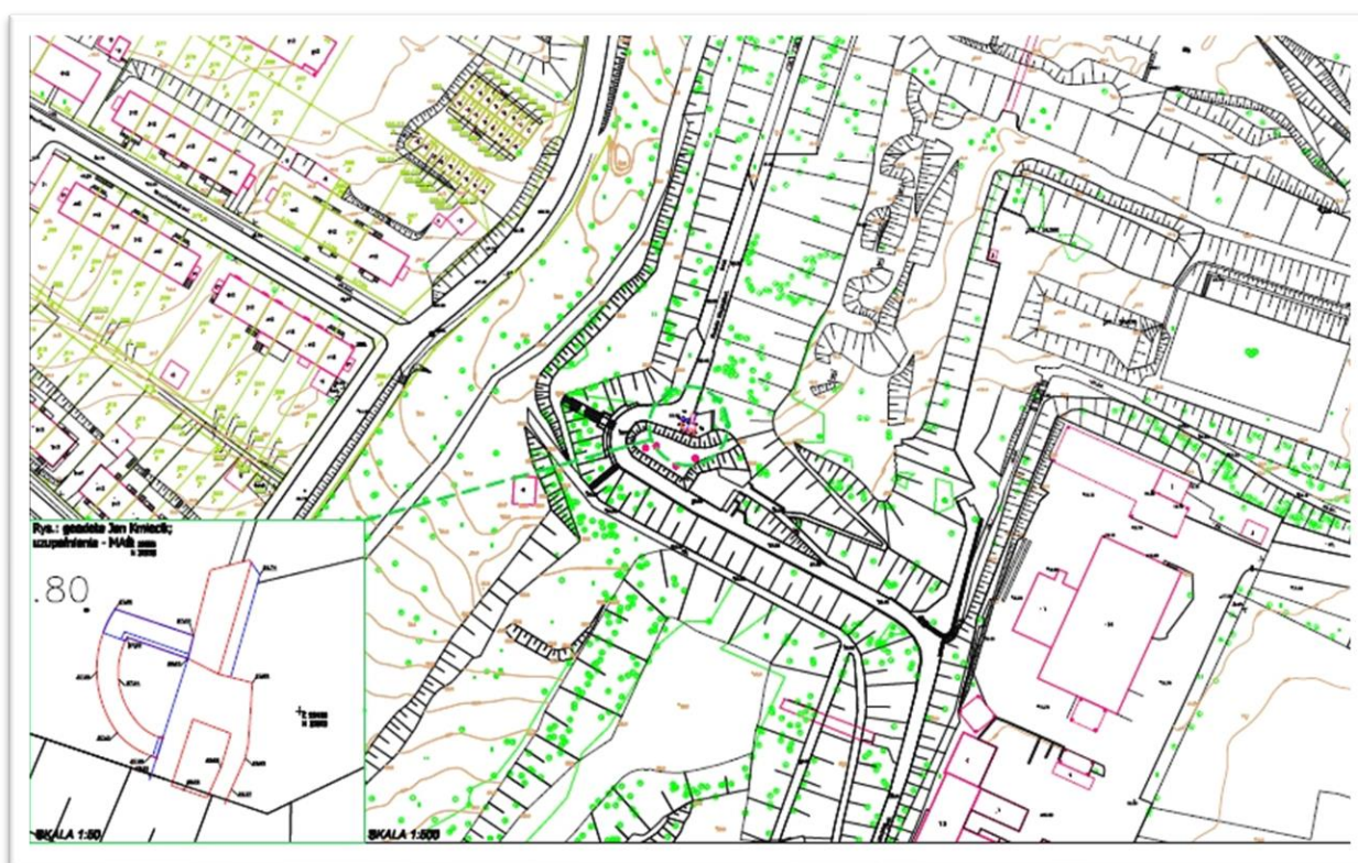
Ryc.5.48 Rzut reliktów Bramy Wschodniej wraz z komorą z mechanizmem mostu zwodzonego i murem przeciwskarpy przy bramie (rysunek wykonany w Pracowni Informatyczno -pomiarowej Muzeum Archeologicznego w Gdańsku)
