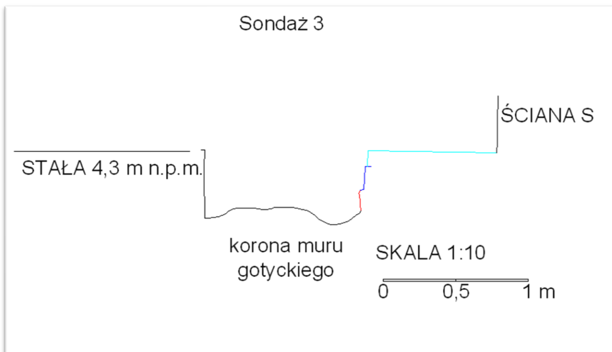
Ryc.2.17 Przekrój przez odsłonięty fragment korony gotyckiego muru zalegającego poniżej muru wschodniego bastei (rys. M. Kasprzak, oprac. Dział Cyfryzacji i Archiwizacji Muzeum Archeologiczne w Gdańsku)
