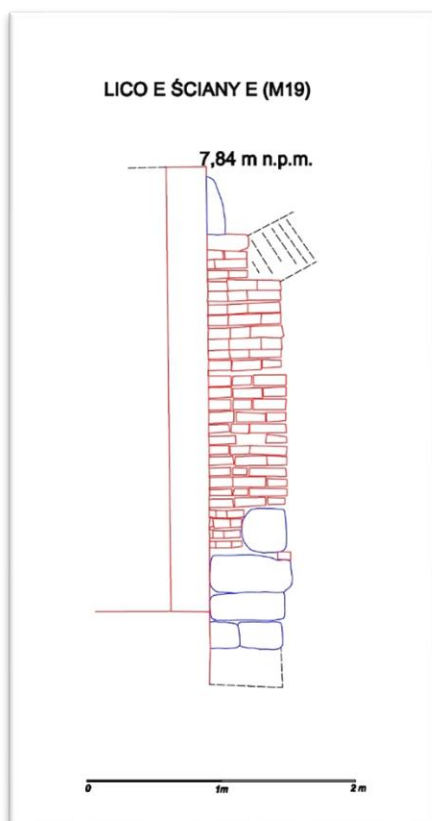
Ryc.4.28 A Fundament przejazdu bramnego wraz z kamieniem wyznaczającym XVII wieczny poziom przejazdu. Linia przerywana oznaczono łęk pod XIX wieczny poziom użytkowy przejazdu (rys. D. Dyduch, oprac. M. Kasprzak), B Fundamenty pod XIX elewację wschodniej ściany Bramy Wyżynnej doklejone do pierwotnego fundamentu przejazdu bramnego. U góry widoczny kamień wyznaczający XVII w poziom użytkowy oraz fragment łuku z cegły maszynowej. Widok od NE (fot. i oprac. M. Kasprzak)
