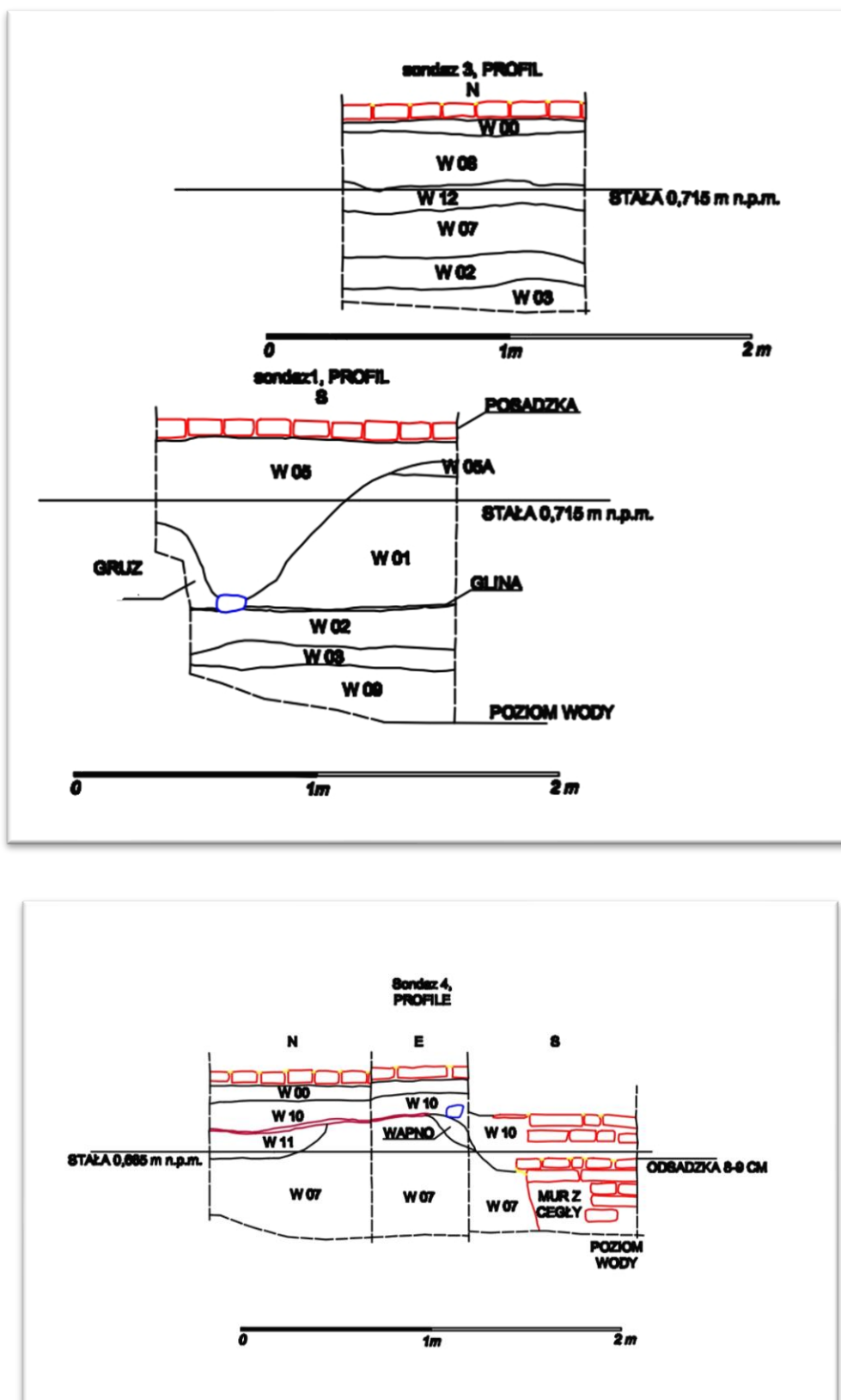
Ryc.6.51 Profile sondażu nr 1,3,4 wewnątrz Bastionu Artyleryjskiego z 2002 roku. Warstwy 02,03,09-okres budowy Fortu Carre, warstwy 01,07,11,12 - niwelacje pod poziom użytkowy 05A z XVII -XVIII wieku, warstwy 10, 05,00 -podnoszenie terenu w latach 70 tych XIX wieku. W sondażu 4 warstwę użytkową z XVII -XVIII wieku oznaczono kolorem czerwonym (rys. A. Nakonieczna, oprac. A. Pudło, M. Kasprzak)
