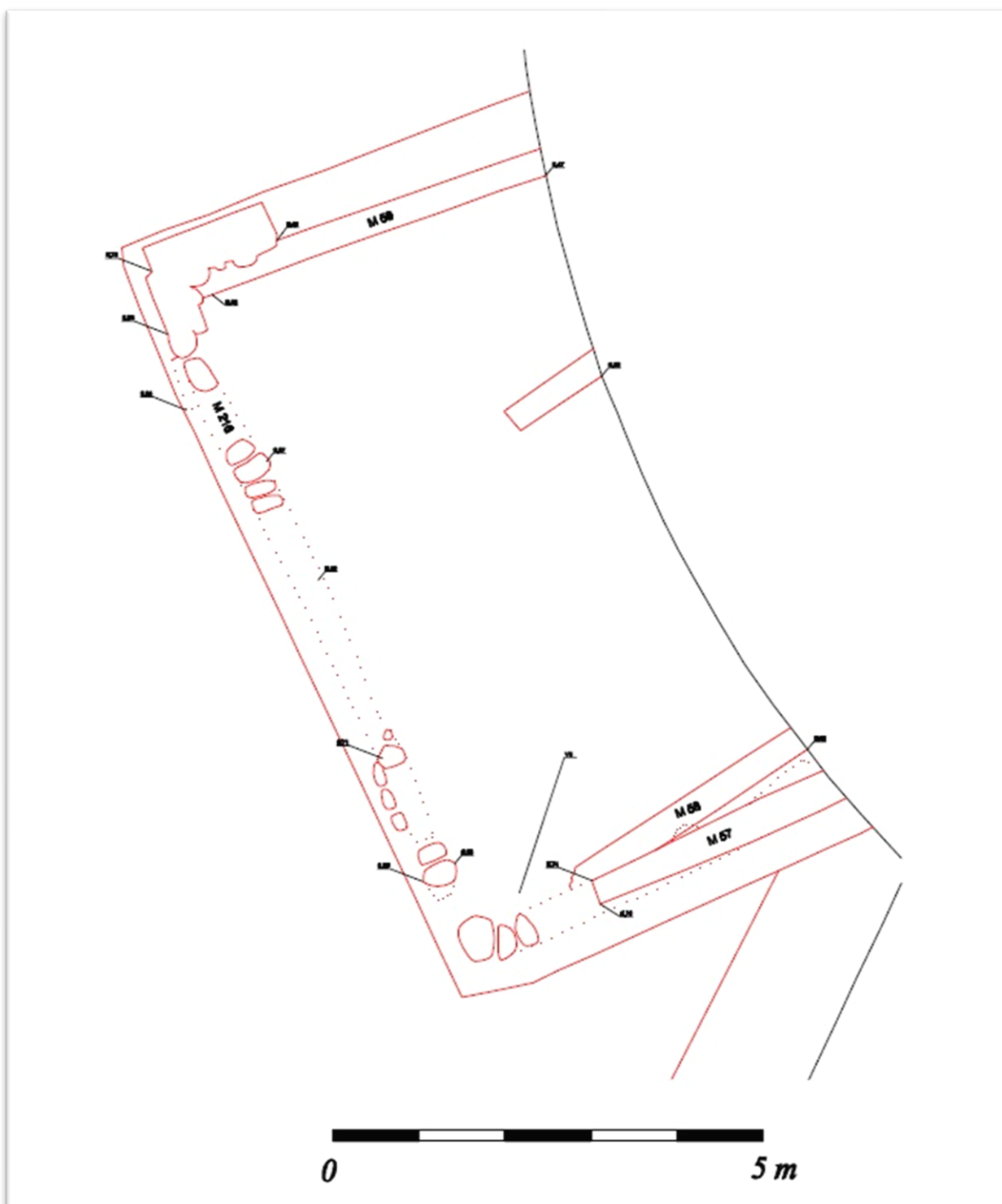
Ryc.6.7 Pozostałości fundamentów XVII -XIX wiecznych prochowni odsłonięte podczas badań w 2003 roku (rysunek i pomiary P. Janda)
