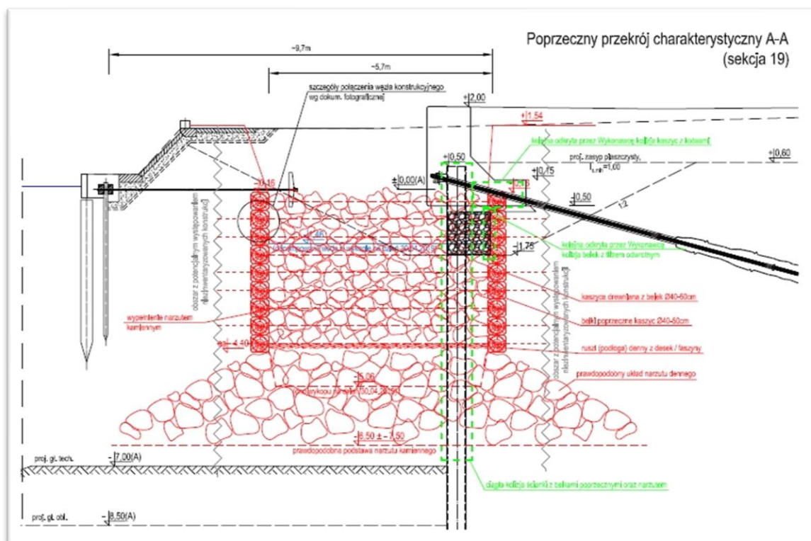
Ryc.6.76 A Przekrój poprzeczny A-A jednej z kaszyc (sekcja19) odkrytych wzdłuż nabrzeża Zbożowego w 2019 roku,
