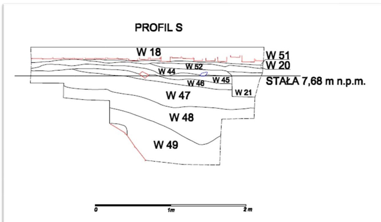
Ryc.4.44 Profil W i S sondażu 2 z 2010 roku. Poniżej współczesnego poziomu użytkowego XIX wieczne nawarstwienia tworzące zasyp fosy. Nawarstwienia miejscami przecięte przez współczesne wkopy (rys. D. Dyduch, oprac. M. Kasprzak)
