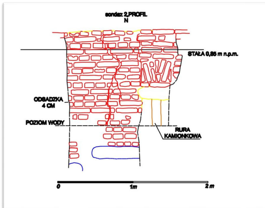
Ryc.6.52 Sondaż 2 z 2002 roku -fragment ściany Bastionu Artyleryjskiego z odpływem syfonu zamontowanego w latach 70 -tych XIX (rys. A. Nakoneczna, oprac. A. Pudło)
