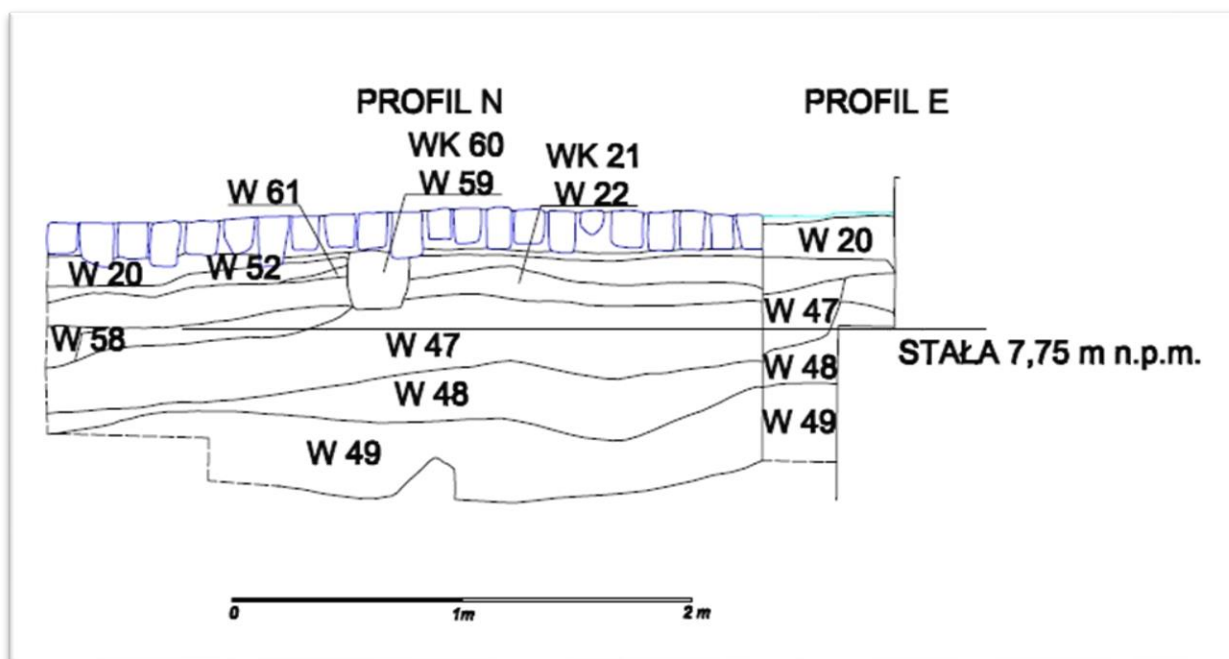
Ryc.4.48 Profil E i S sondażu 3 z 2010 roku. Poniżej współczesnego poziomu użytkowego XIX wieczne nawarstwienia tworzące zasyp fosy. Nawarstwienia miejscami przecięte przez współczesne wkopy (rys. D. Dyduch, oprac. M. Kasprzak)
