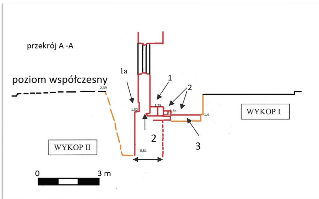
Ryc. 3.39 C Przekrój przez wykopy na osi N- S w obrębie wschodniej wartowni Bramy Nizinnej. Cyfrą 1 oznaczono wewnętrzną odsadzkę muru, 1A zewnętrzną odsadzkę, cyfrą 2 fragment posadzki, cyfra 3 - rurę kanalizacyjną (rys. i oprac. A. Pudło)
