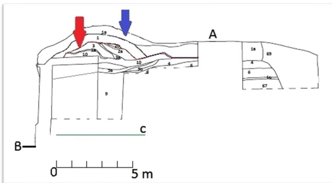
Ryc.6.9 Profil N wykopu I z 2003 roku w części północnej kurtyny zachodniej. A - współczesny poziom użytkowy, B - poziom wody 0 m. n. p. m, C domniemany poziom użytkowy działobitni z przełomu XVI i XVII wieku. Strzałką czerwoną oznaczono poziom XVII wiecznego nasypu. Strzałką niebieską oznaczono poziom nasypu w XIX wieku (rys. B. Balewska, oprac. M. Schmidt)
