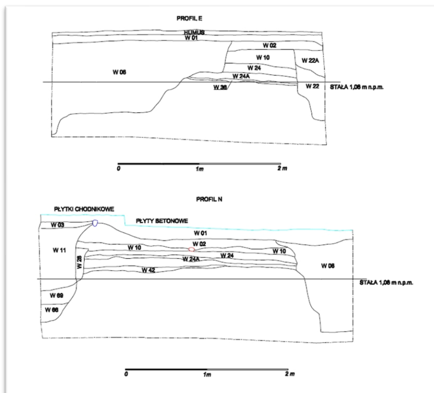
Ryc.6.56 Profil N i E sondażu I założonego w 2000 przy Domkach Oficerskich. Z okresu po 1945 roku pochodzą humus, betonowe płyty, podsypka pod nie (w.01), wkop pod ścianę domu powstały w latach 70 tych XX wieku (w.03,11), z remontem z lat 70 tych XIX wieku łączyć wkop pod kanalizację burzową (w.08), niwelacje podnoszące teren (w.02), z XVIII wieku pochodzi warstwa budowlana (w.10) oraz pozostałości wkopu naprawczego (?) pod domek (w.28) , z XVII wieku pochodzi warstwa użytkowa (w.24, 24A) i piaskowa podsypka (w.36) oraz pozostałości pierwotnego wkopu pod domek (66,69), najstarszy poziom użytkowy z przełomu XVI i XVII wieku ( w.42) (rys. L. Lotkowski, oprac. A. Pudło, M. Kasprzak)
