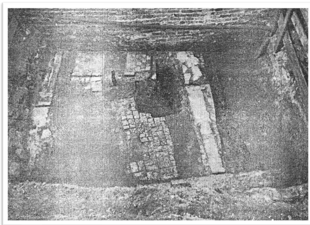
Ryc.6.6 Pozostałości fundamentów XVII -XIX wiecznych prochowni usytuowanych przy zachodniej ścianie Wieńca (Zbierski 1977, s.136, rys.3, wykop VIII)
