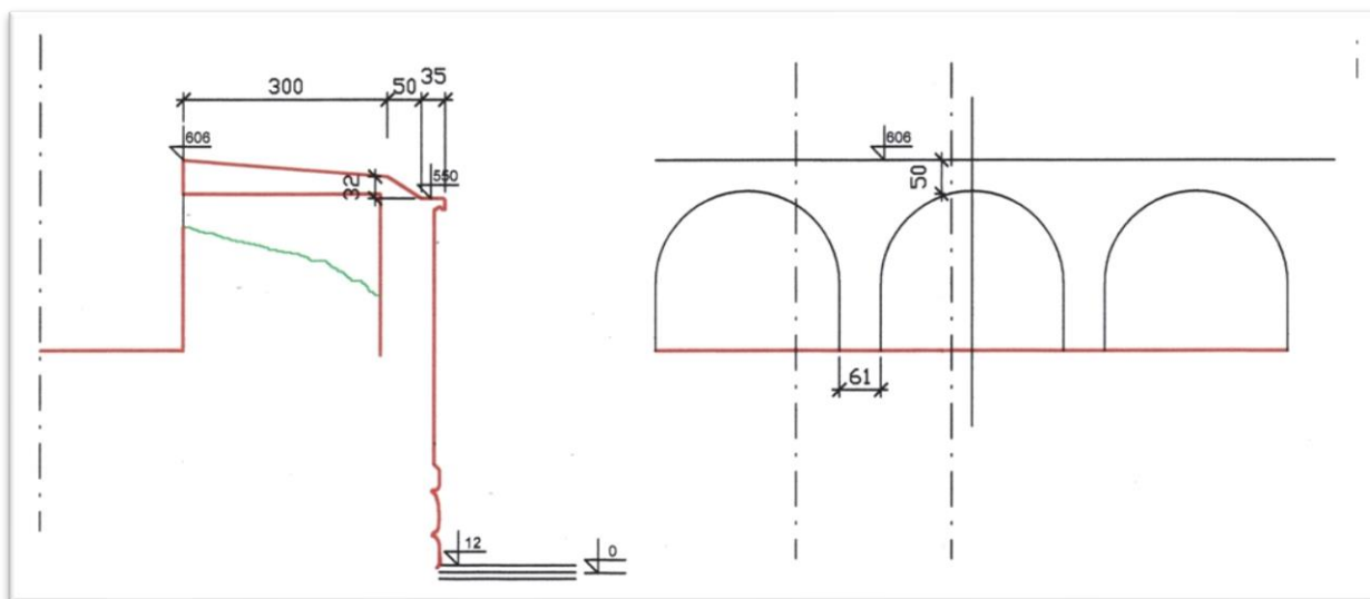
Ryc.6.11 Przekrój przez odkryta działobitnię i rekonstrukcja trzech działobitni umieszczonych w murze zachodnim Fortu Carre (rys. i oprac G. Bukal)
