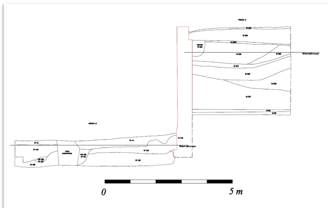
Ryc.6.35 Przekrój przez północną ścianę Domu Porucznika Piechoty (obecnie pełniące funkcję muru oporowego) oraz nawarstwienia ziemne dolegające bezpośrednio do niego (rys. B. Balewska, oprac. M. Kasprzak)
