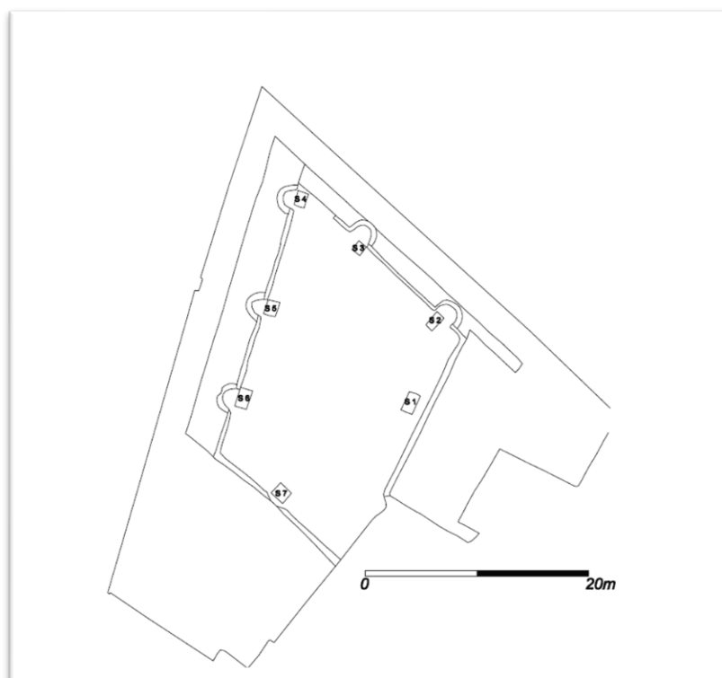
Ryc.6.50 A. Rzut Bastionu Artyleryjskiego z zaznaczonymi sondażami z 2001 i 2002 roku (rys. A. Nakonieczna, oprac. A. Pudło)
