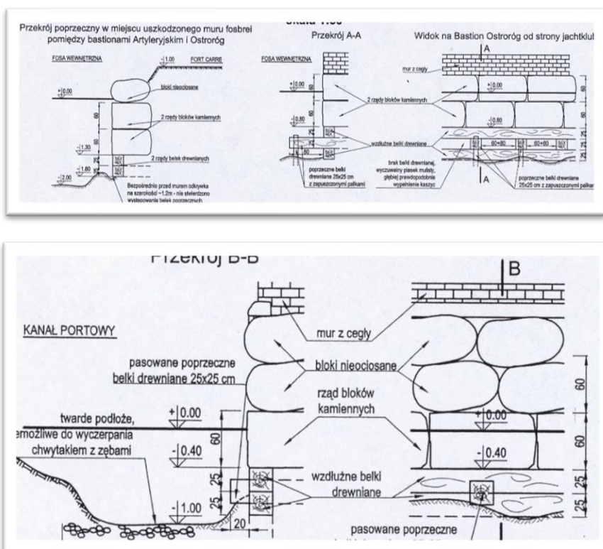
Ryc.6.69 Fundamenty Bastionu Ostroróg, Artyleryjskiego oraz muru fosbrei wykonane od strony fosy i ujścia Wisły (oprac. Cz. Goszek)
