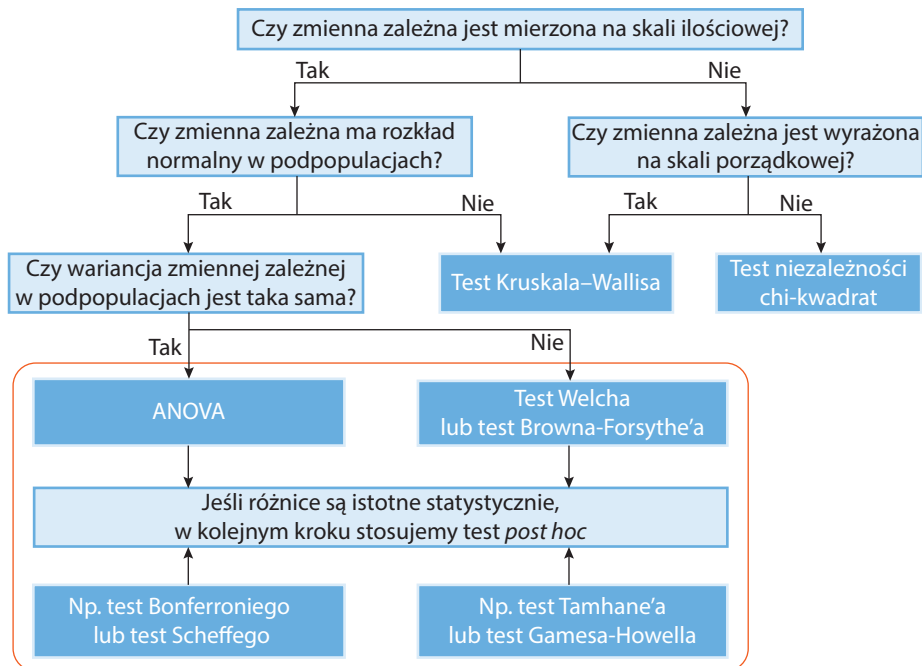
Rysunek 2.2. Schemat wyboru testu przy porównaniu przynajmniej dwóch populacji – pomiar niezależny
