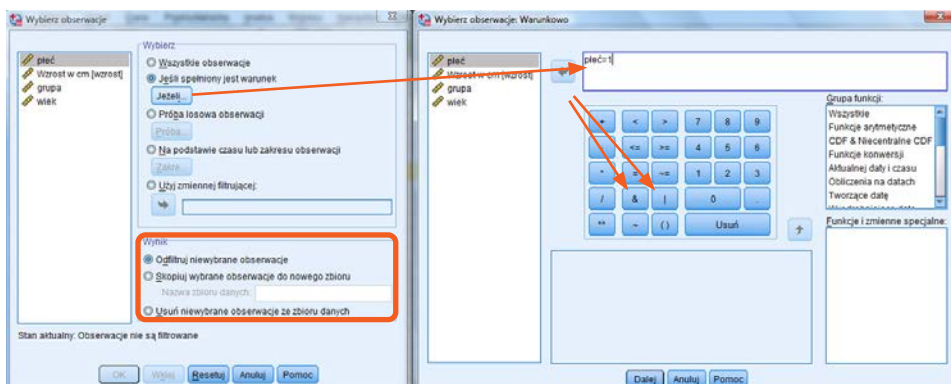
Rysunek 1.19. Wykonywanie polecenia Wybierz obserwacje – wybór podpróby według wskazanych kryteriów
