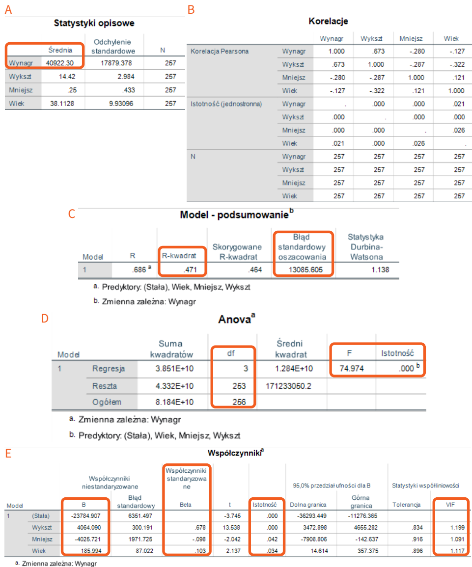
Rysunek 7.7. Wyniki estymacji modelu wynagrodzeń: y = f(\text{Wyksz}, \text{Wiek}, \text{Mniejszy})
