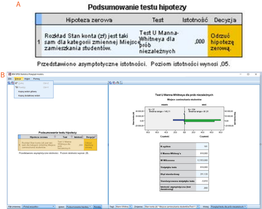
Rysunek 4.9. Wyniki analiz testem Manna-Whitneya (ścieżka 2)
