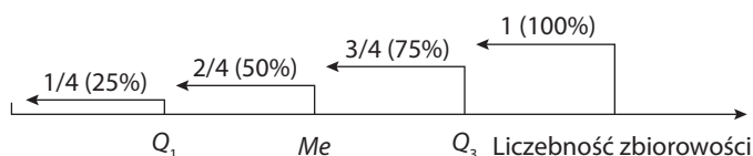
Rysunek 3.4. Podział zbiorowości statystycznej na kwantyle
