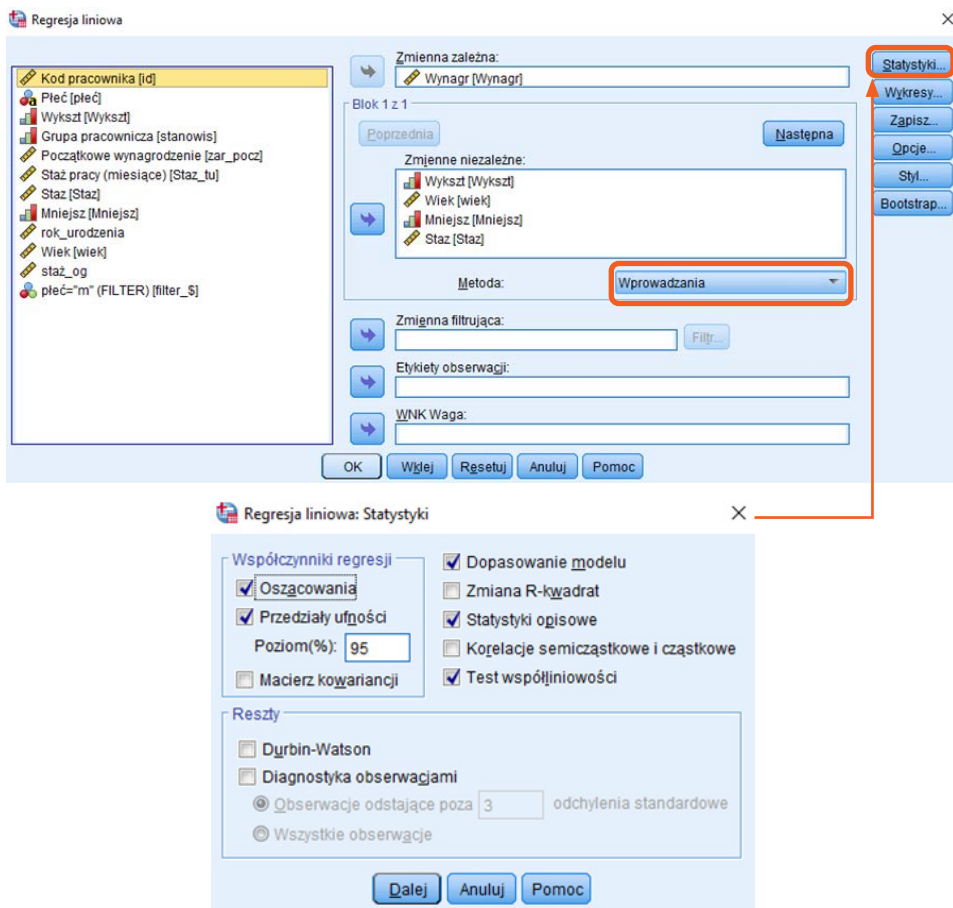
Rysunek 7.5. Okno polecenia Regresja liniowa – estymacji modelu wynagrodzeń: y = f(\text{Wyksz}, \text{Wiek}, \text{Mniejsz}, \text{Staz})
