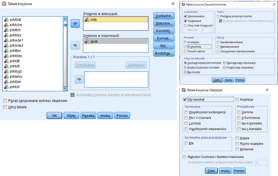
Rysunek 6.1. Wykonywanie polecenia Tabele krzyżowe
