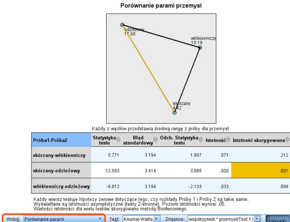
Rysunek 5.13. Widok okna raportowego z wynikami porównań wielokrotnych: porównanie zmiennej wsk według przemysł (ścieżka 2)
