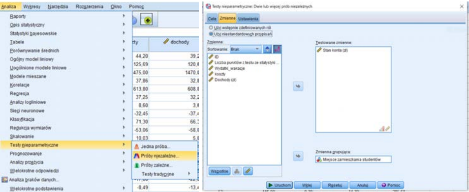
Rysunek 4.8. Wykonywanie testu Manna-Whitneya (ścieżka 2)
