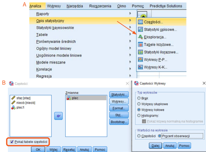
Rysunek 3.1. Wykonywanie polecenia Częstości
