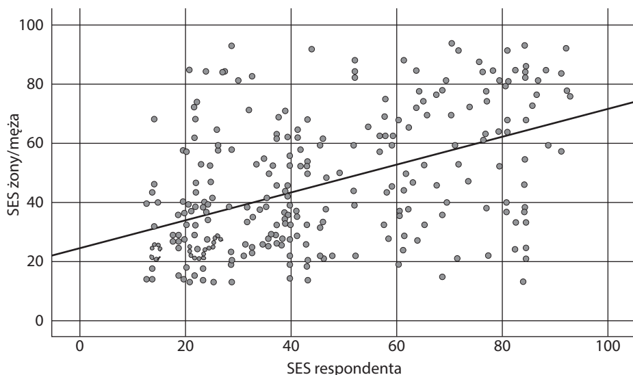
Rysunek 6.18. Wykres rozrzutu/punktowy dla zmiennych SEI10 i SPSEI10
