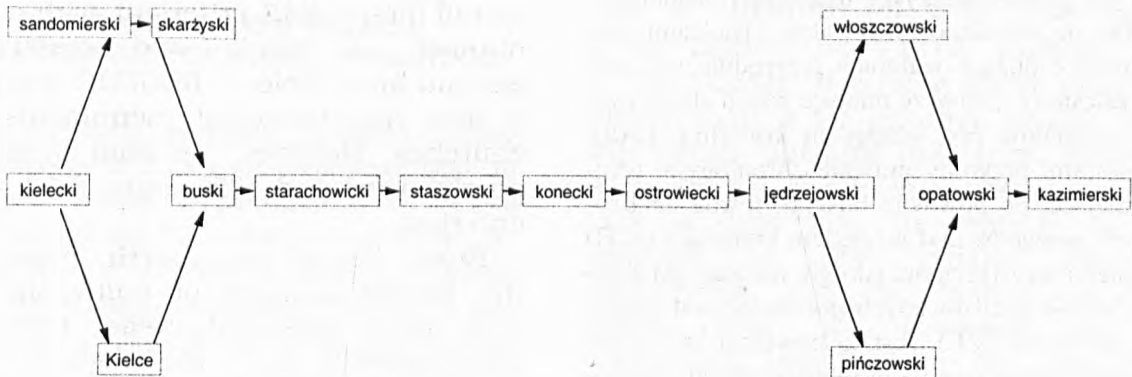
Rys. 5. Graf porządku częściowego analizy powiatów województwa świętokrzyskiego (ź r ó d ł o: opracowanie własne przy wykorzystaniu programu Promcalc & Gaia )
