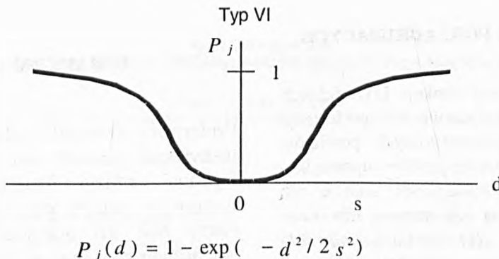
Rys. 3. Model „ciągły” analizy preferencji (źródło: BRANS, MARESCHAL 1994, BRANS, MARESCHAL 1990)
