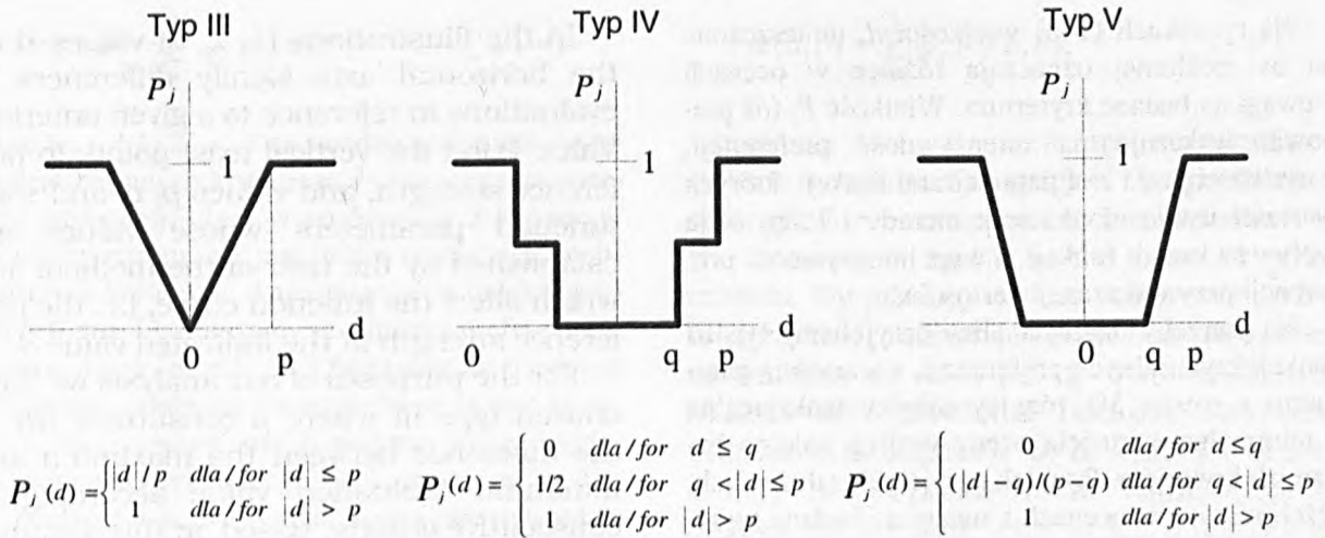
Rys. 2. Modele ze stopniowaniem odczuć preferencji (źródło: BRANS, MARESCHAL 1994, BRANS, MARESCHAL 1990)
